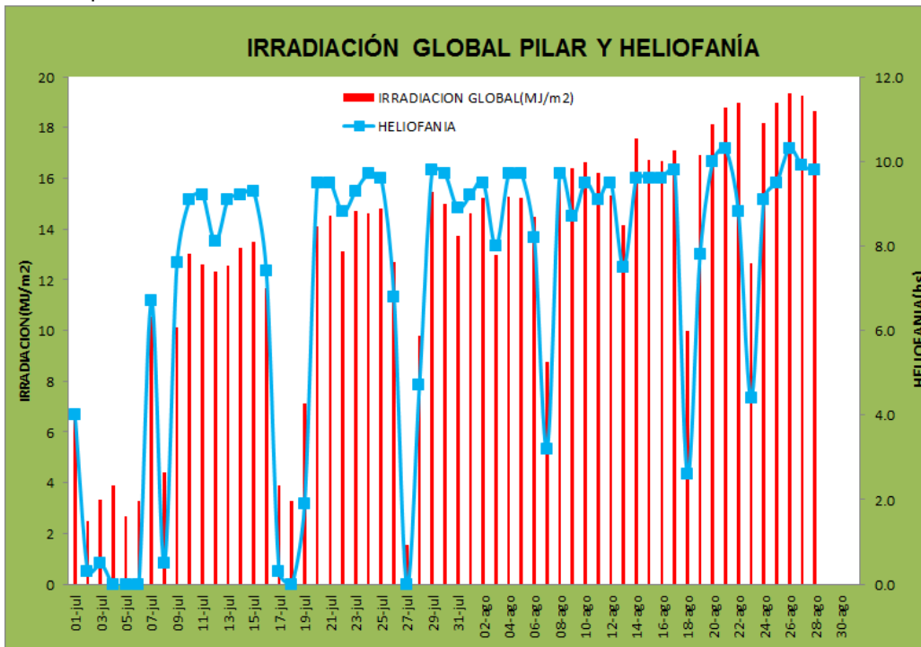
Figura 17. Heliofanía efectiva diaria junto con irradiación solar global diaria, ambas para la ciudad de Pilar.
