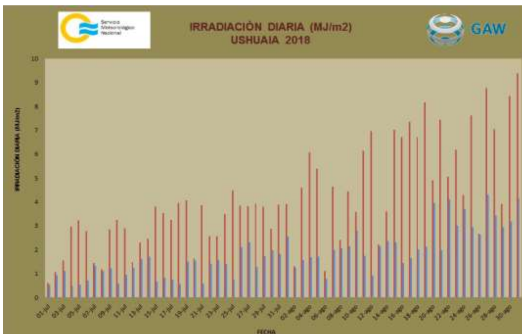
Figura 12. Irradiación global y difusa medida en Ushuaia.
