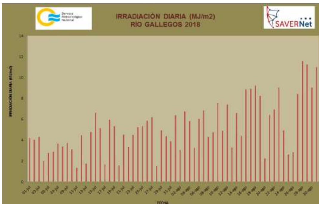
Figura 10. Irradiación global medida en Río Gallegos.
