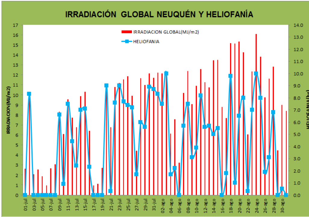
Figura 16. Heliofanía efectiva diaria junto con irradiación solar global diaria, ambas para la ciudad de Neuquén.
