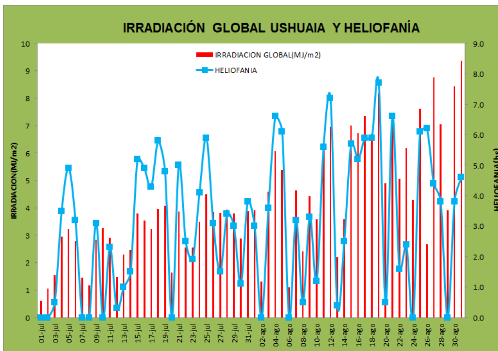
Figura 20. Heliofanía efectiva diaria junto con irradiación solar global diaria, ambas para la ciudad de Ushuaia.
