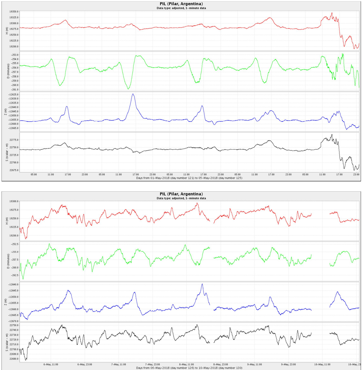
Figura 4a: Componentes del campo magnético del 1 al 10 de Mayol. En rojo se ve la componente horizontal (H) y en azul la vertical (Z), ambas en nT. En verde se presenta la declinación del campo magnético (D) en minutos y en negro la intensidad del campo magnético en nT
