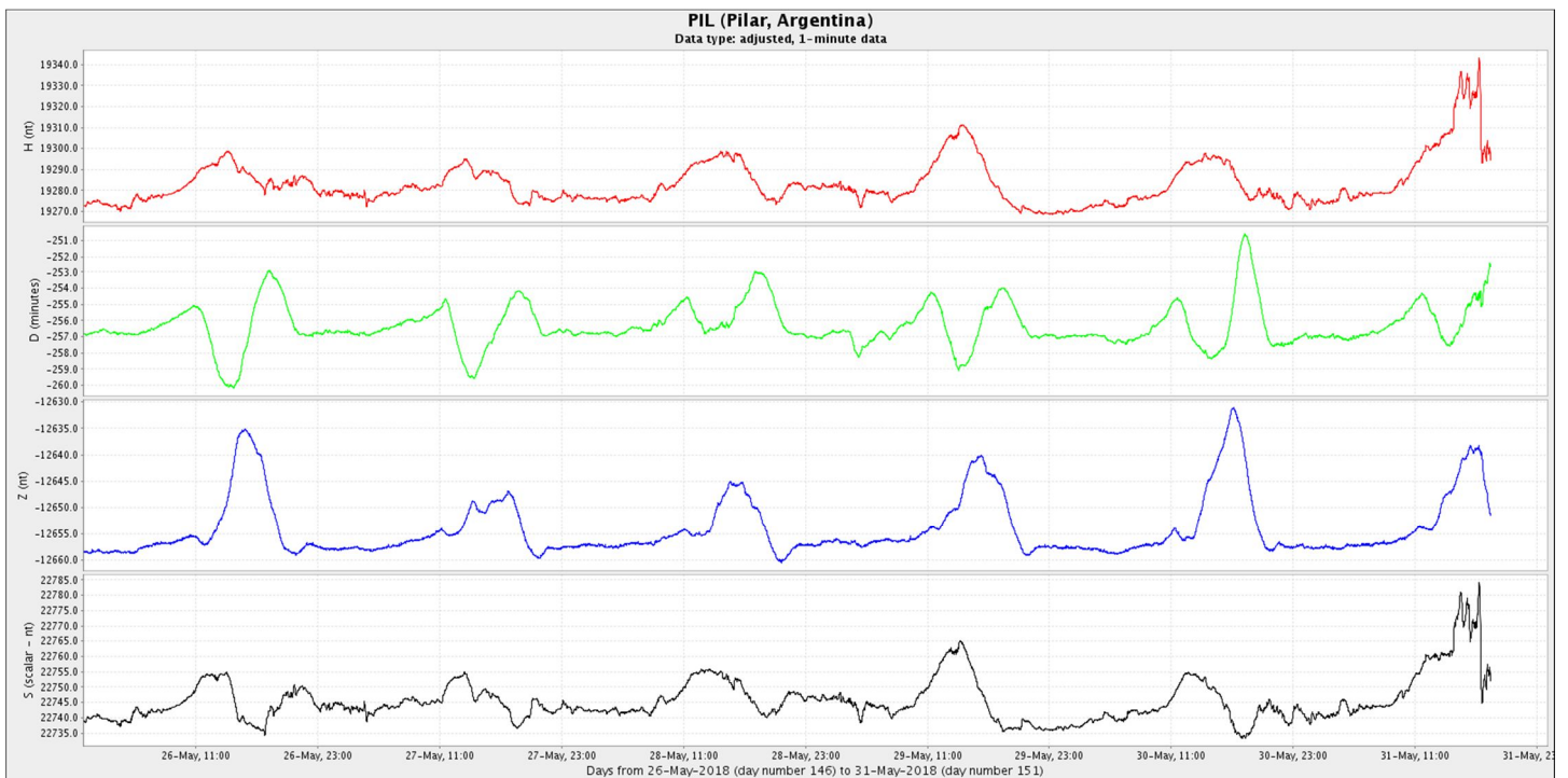
Figura 4c: Componentes del campo magnético del 21 al 31 de Mayo.. En rojo se ve la componente horizontal ( H ) y en azul la vertical ( Z ), ambas en nT. En verde se presenta la declinación del campo magnético ( D ) en minutos y en negro la intensidad del campo magnético en nT.
