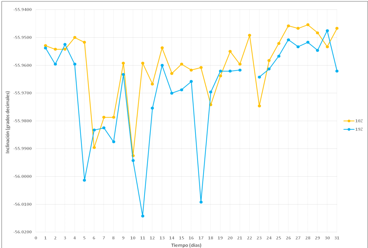
Figura 6: Inclínación magnética en función del tiempo
