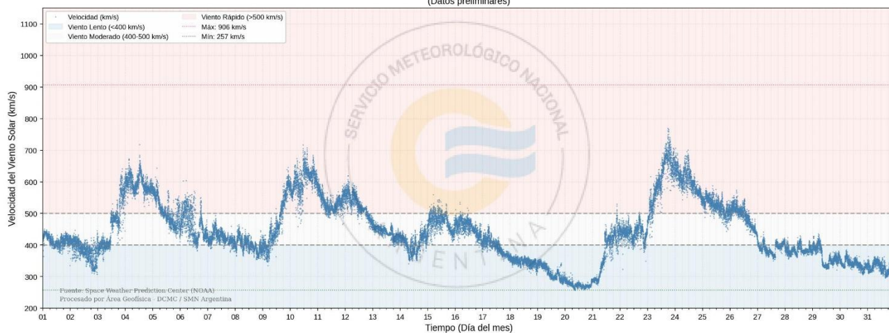
Figura 7: Evolución del viento solar durante el mes de Julio de 2026 (Datos provisionales)
