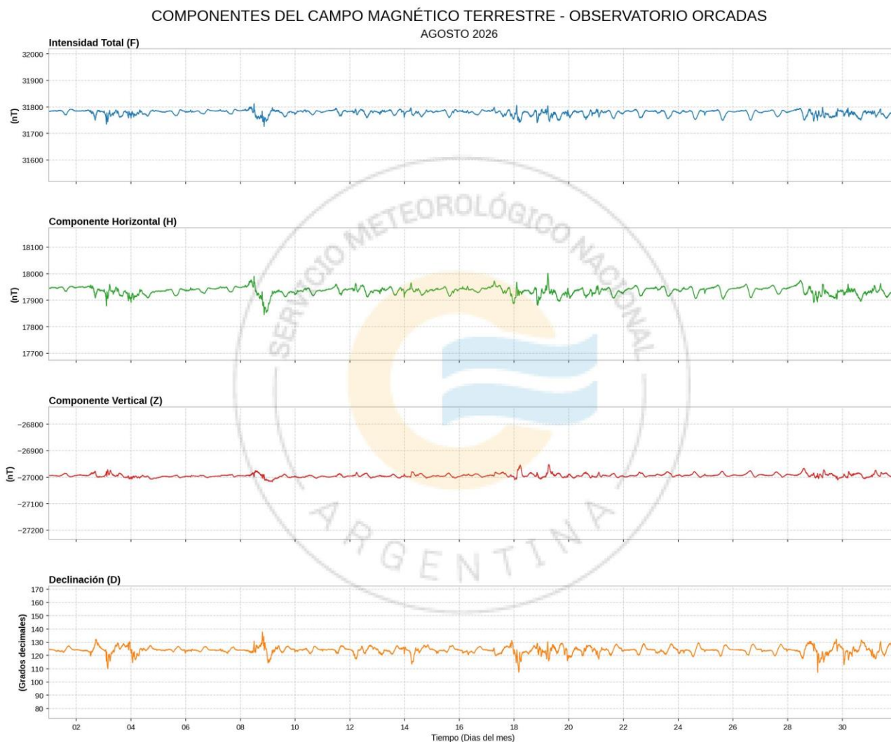
Figura 3: Componentes del campo magnético durante el mes de Agosto de 2026. En azul la intensidad del campo magnético (F), en verde la componente horizontal (H) y en rojo la componente vertical (Z), todas medidas en nanoteslas (nT). En naranja se presenta la declinación del campo magnético (D) expresada en decimas de grado.
