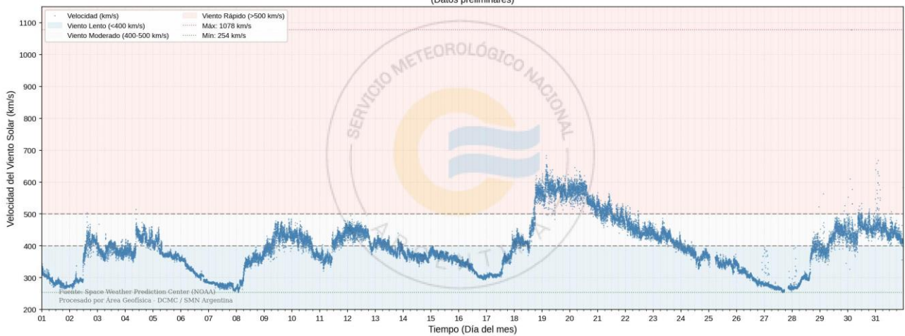
Figura 7: Evolución del viento solar durante el mes de Agosto de 2026 (Datos preliminares)
