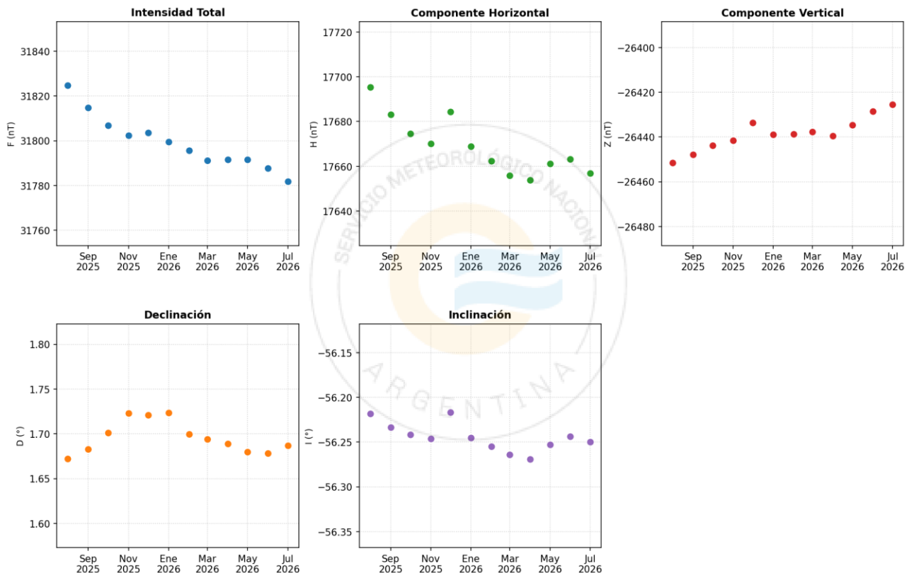
Figura 5: Valores medios mensuales de los elementos absolutos del campo magnético medidos en el observatorio durante los últimos 12 meses. F , H y Z están expresadas en nanotesla (nT); D e I en grados decimales (°)
