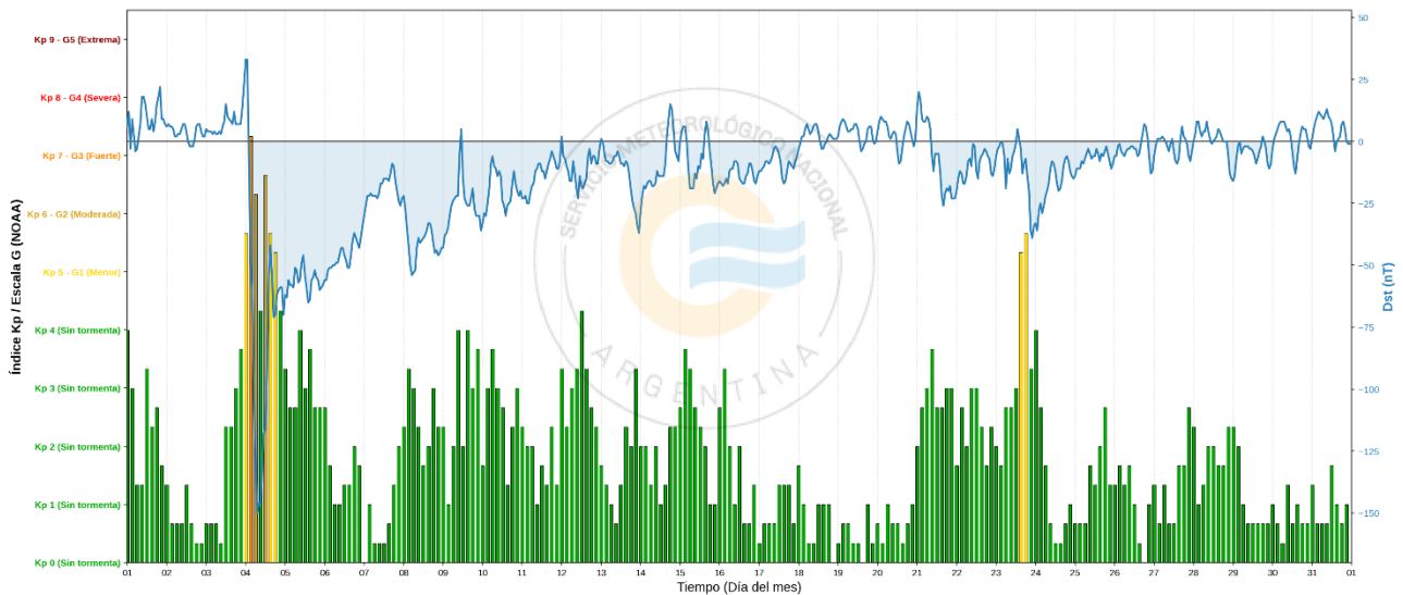
Figura 6: Evolución de la actividad geomagnética global durante el mes de Julio de 2026. Índices Kp y DST son provisionales
