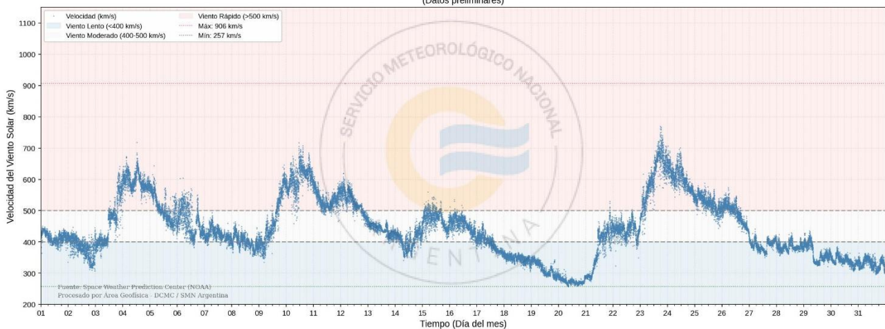
Figura 7: Evolución del viento solar durante el mes de Julio de 2026 (Datos preliminares)
