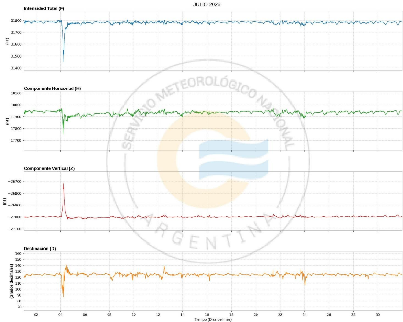
Figura 3: Componentes del campo magnético durante el mes de Julio de 2026. En azul la intensidad del campo magnético (F), en verde la componente horizontal (H) y en rojo la componente vertical (Z), todas medidas en nanoteslas (nT). En naranja se presenta la declinación del campo magnético (D) expresada en decimas de grado.
