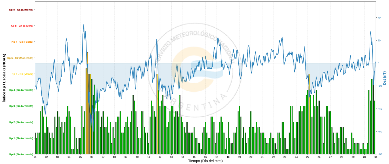
Figura 6: Evolución de la actividad geomagnética global durante el mes de junio de 2026 (Índices Kp y DST son provisionales)
