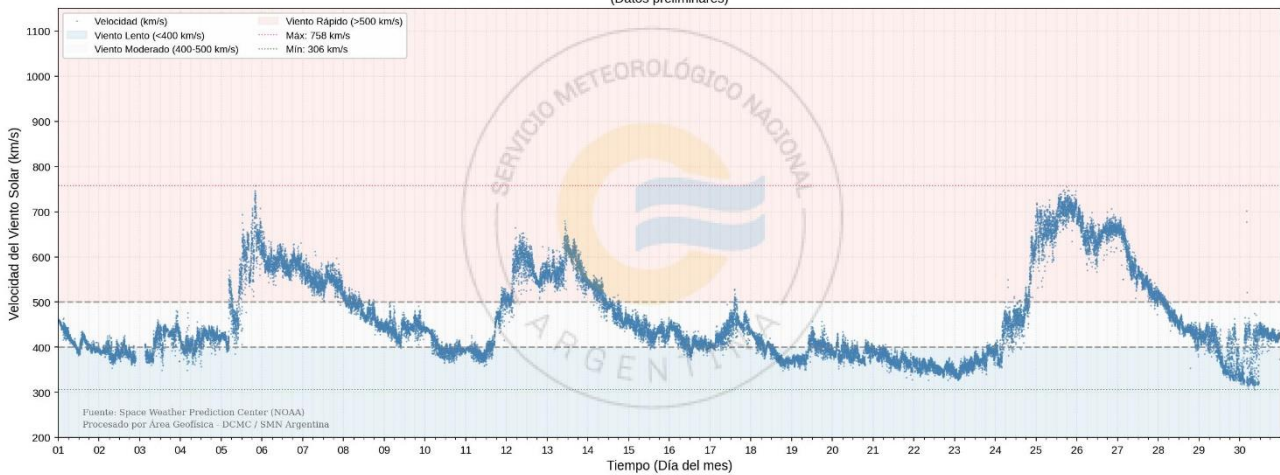
Figura 7: Evolución del viento solar durante el mes de junio de 2026 (Datos provisionales)
