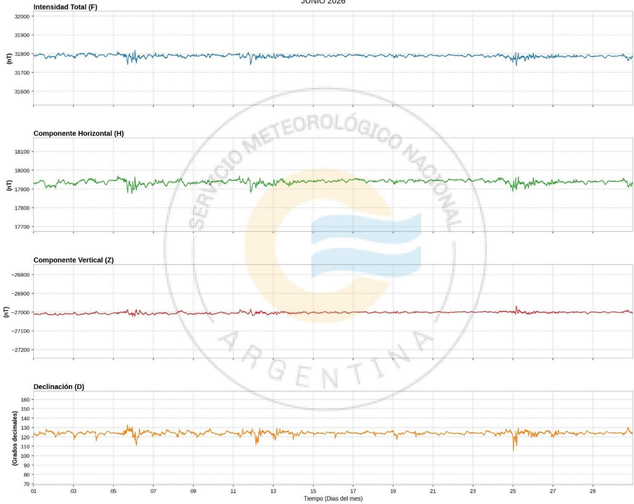
Figura 3: Componentes del campo magnético durante el mes de junio de 2026. En azul la intensidad del campo magnético (F), en verde la componente horizontal (H) y en rojo la componente vertical (Z), todas medidas en nanoteslas (nT). En naranja se presenta la declinación del campo magnético (D) expresada en decimas de grado.
