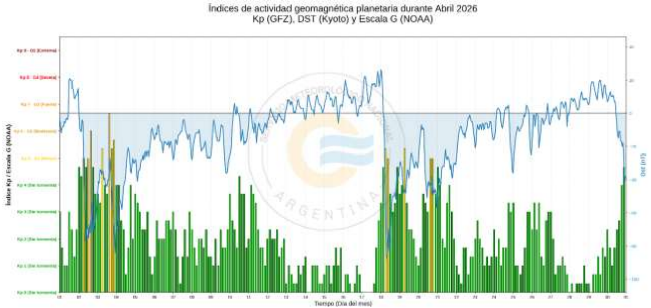
Figura 6: Evolución de la actividad geomagnética global durante el mes de Abril de 2026 (Índices Kp y DST son provisionales)
