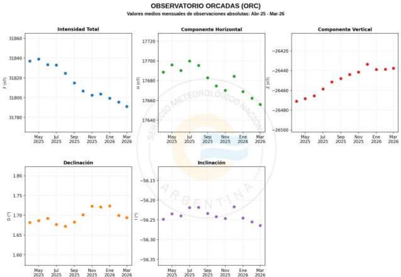
Figura 5: Valores medios mensuales de los elementos absolutos del campo magnético medidos en el observatorio durante los últimos 12 meses. F, H y Z están expresadas en nanoteslas (nT); D e I en grados decimales (°)
