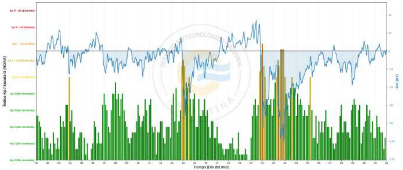
Figura 6: Evolución de la actividad geomagnética global durante el mes de Marzo de 2026 (Índices Kp y DST son provisionales)
