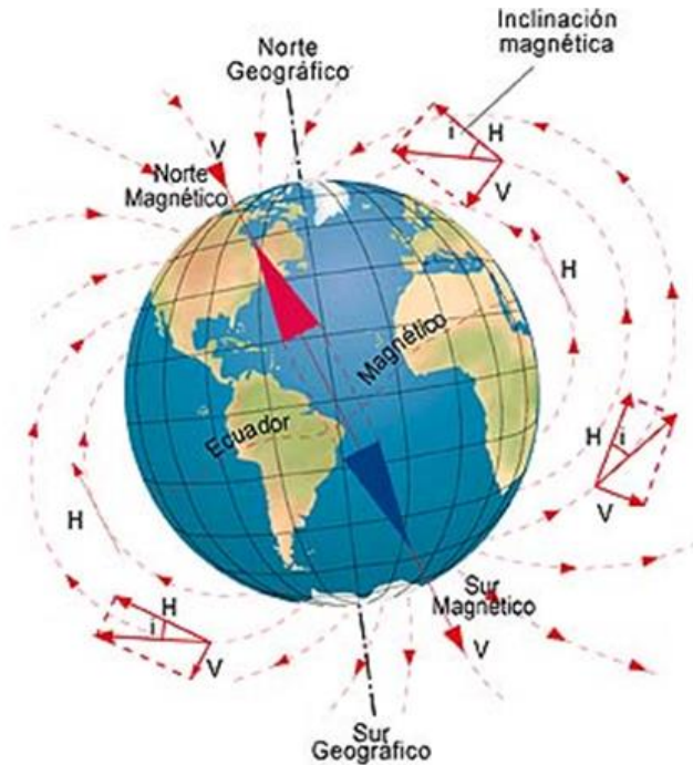
Figura 2: Representación gráfica del campo magnético terrestre
