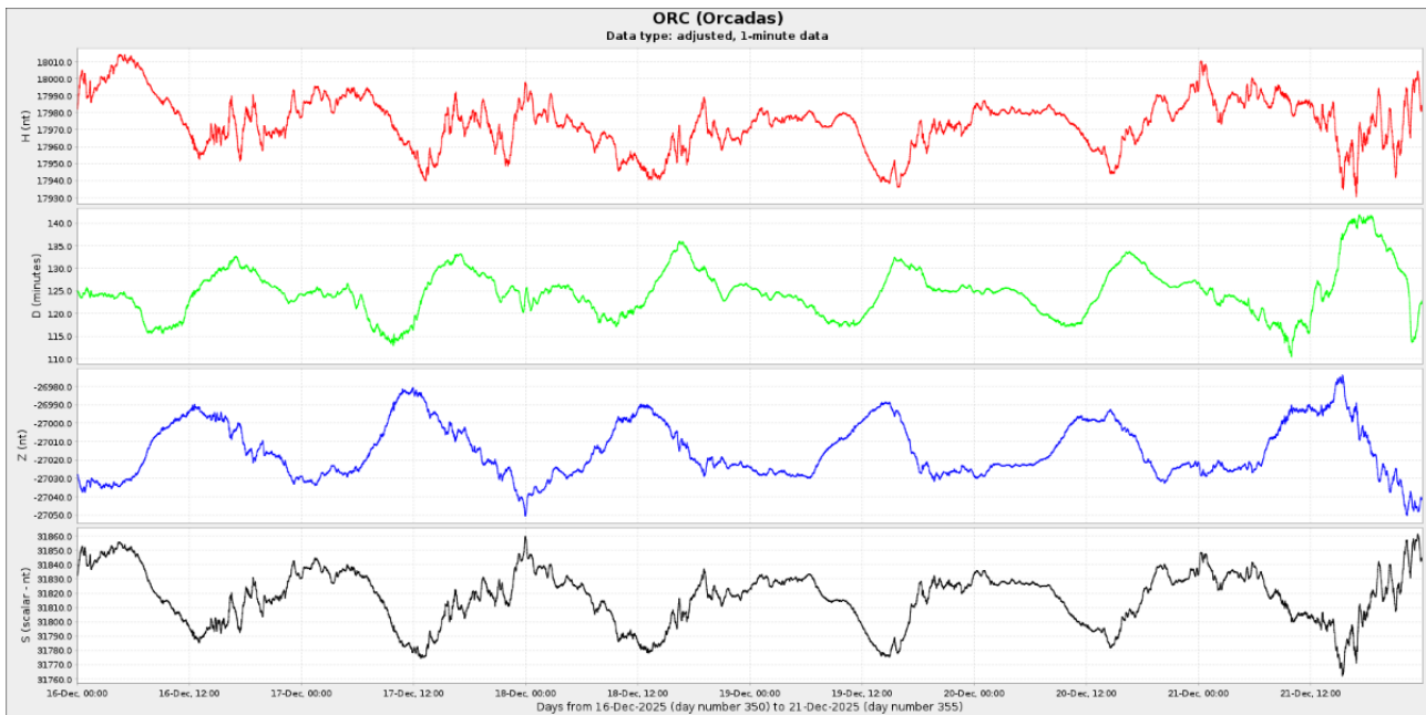
Figura 4b Componentes del campo magnético del 11 al 21 de diciembre. En rojo se ve la componente horizontal (H) y en azul la vertical (Z), ambas en nT. En verde se presenta la declinación del campo magnético (D) en minutos y en negro la intensidad del campo magnético en nT.
