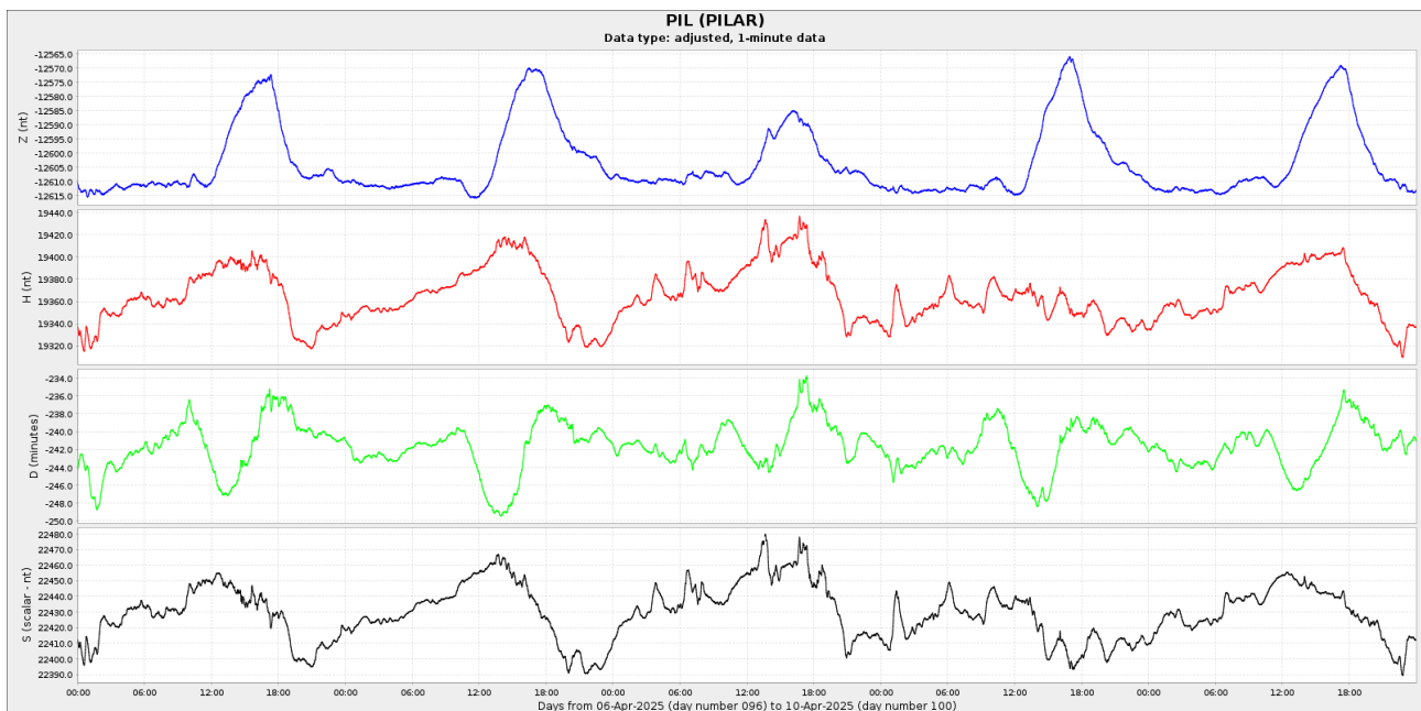
Figura 4a: Componentes del campo magnético del día 1 al 10 de abril. En rojo se ve la componente horizontal (H) y en azul la vertical (Z), ambas en nT. En verde se presenta la declinación del campo magnético (D) en minutos y en negro la intensidad del campo magnético en nT.
