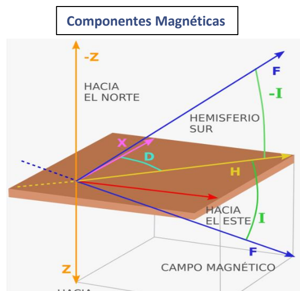
Figura 3: Componentes del campo magnético
