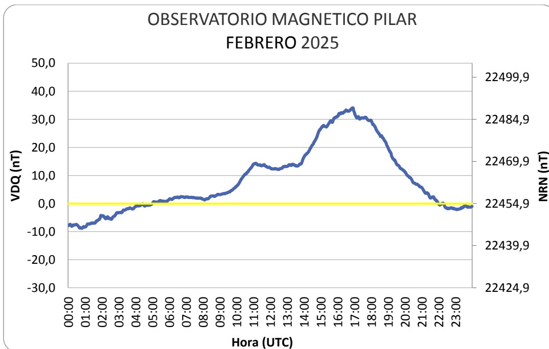
Figura 8: Variación Diaria Calma del mes de febrero
