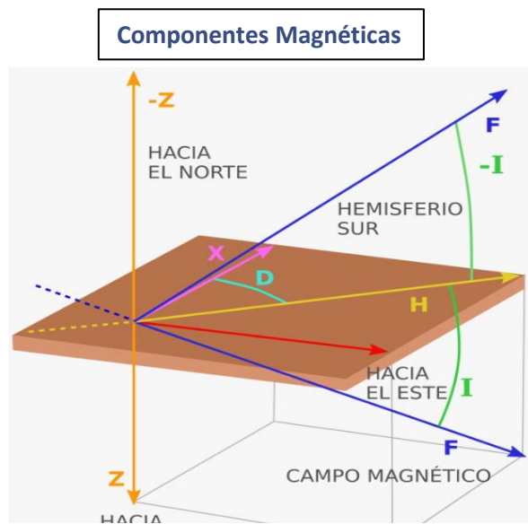
Figura 3: Componentes del campo magnético
