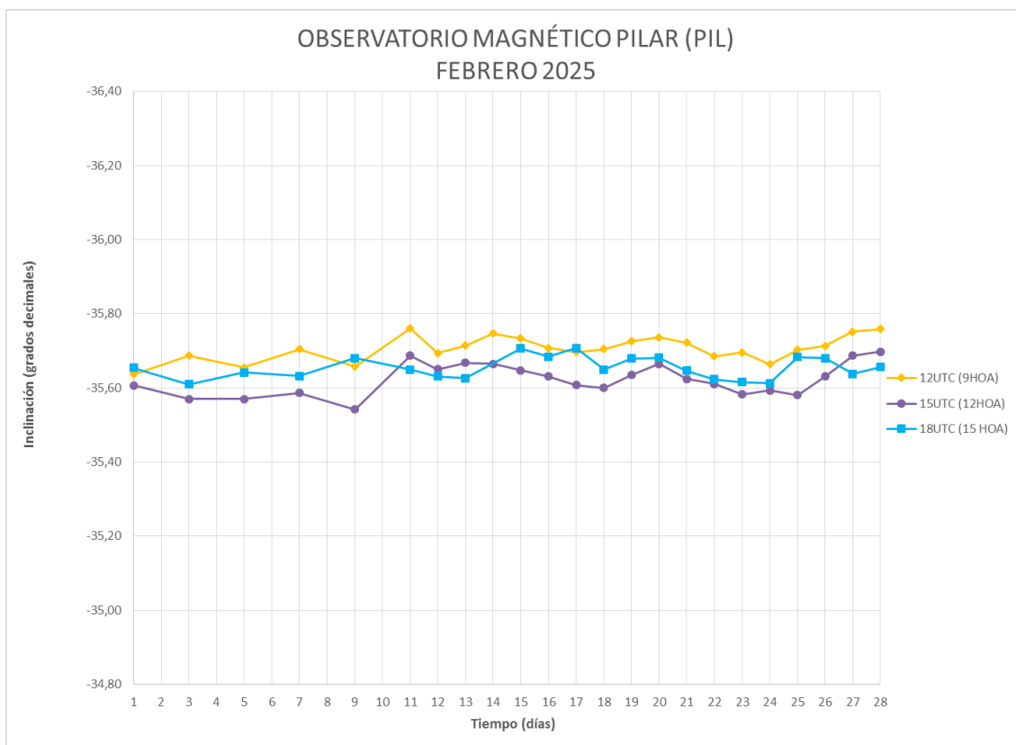
Figura 6: Inclinación magnética en función del tiempo
