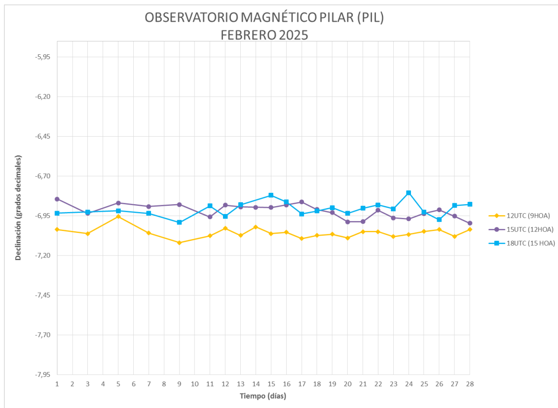
Figura 5: Declinación magnética en función del tiempo
