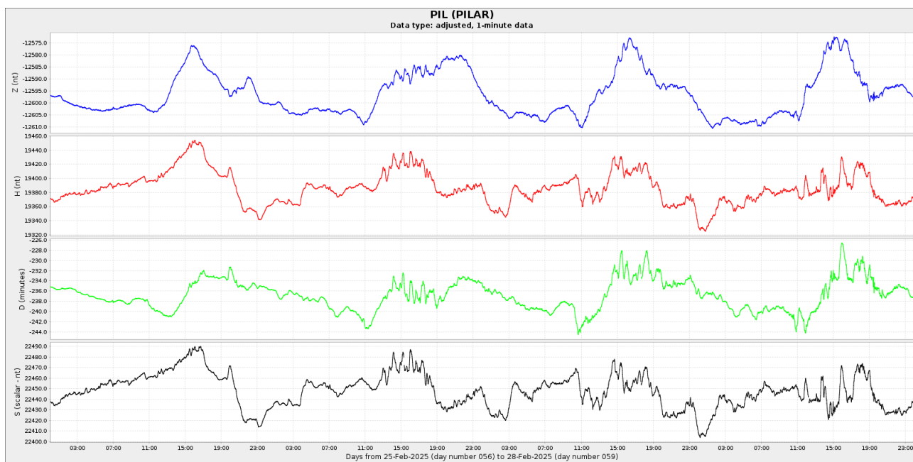
Figura 4c: Componentes del campo magnético del 22 al 28 de febrero. En rojo se ve la componente horizontal (H) y en azul la vertical (Z), ambas en nT. En verde se presenta la declinación del campo magnético (D) en minutos y en negro la intensidad del campo magnético en nT.
