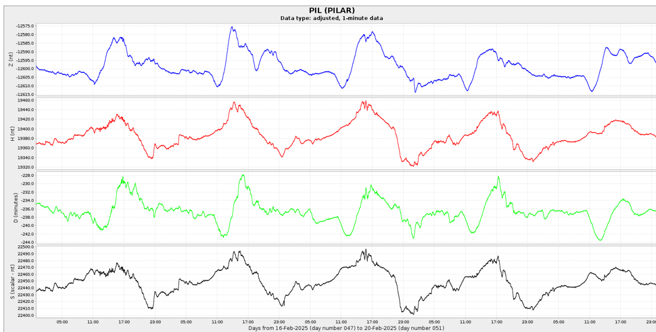
Figura 4b: Componentes del campo magnético del 11 al 21 de febrero. En rojo se ve la componente horizontal ( H ) y en azul la vertical ( Z ), ambas en nT. En verde se presenta la declinación del campo magnético ( D ) en minutos y en negro la intensidad del campo magnético en nT.
