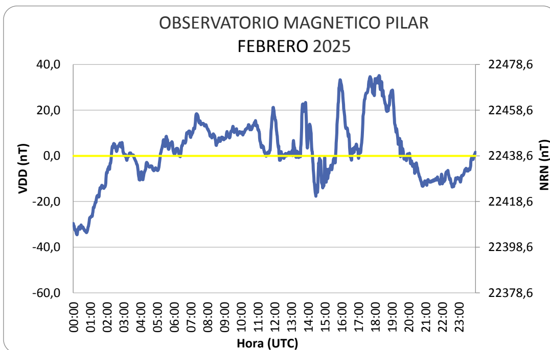
Figura 9: Variación Diaria Perturbada del mes de febrero
