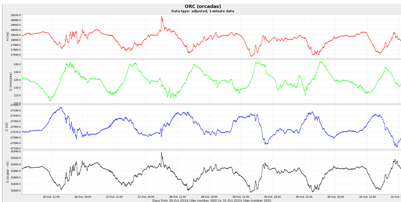
Figura 4c: Componentes del campo magnético del 21 al 31 de octubre. En rojo se ve la componente horizontal ( H ) y en azul la vertical ( Z ), ambas en nT. En verde se presenta la declinación del campo magnético ( D ) en minutos y en negro la intensidad del campo magnético en nT.
