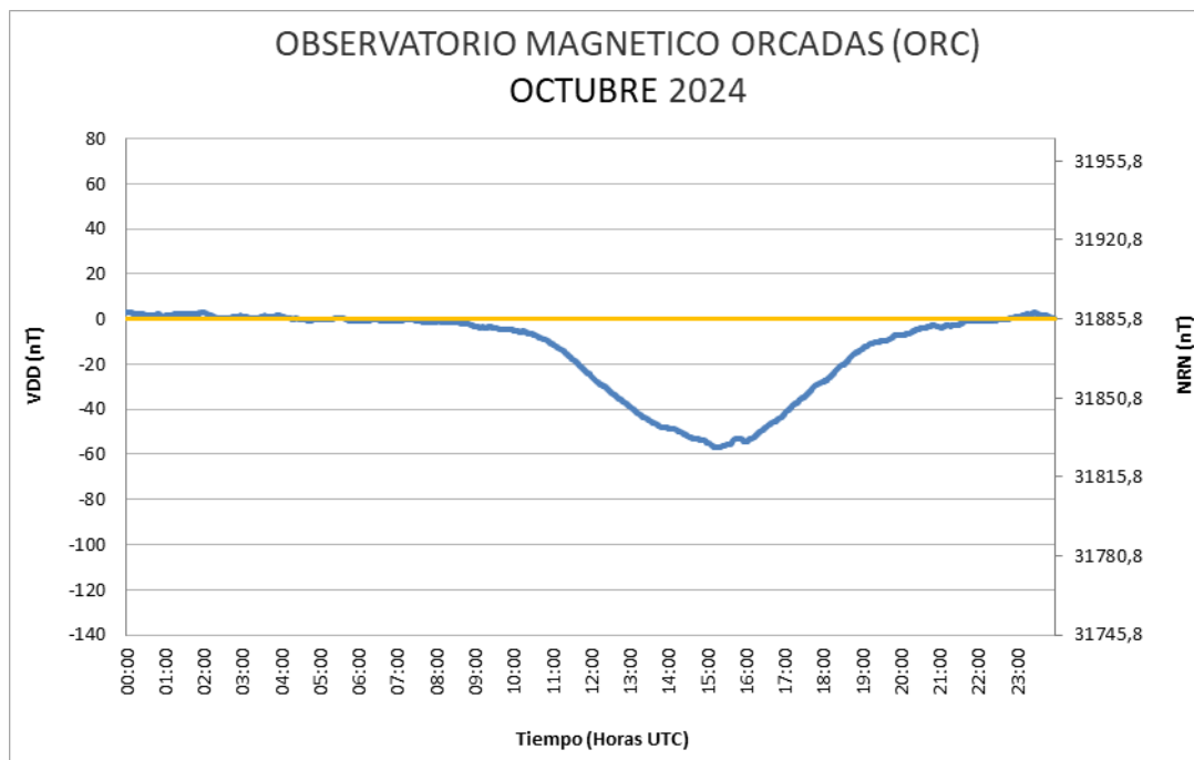
Figura 8: Variación Diaria Calma del mes de octubre
