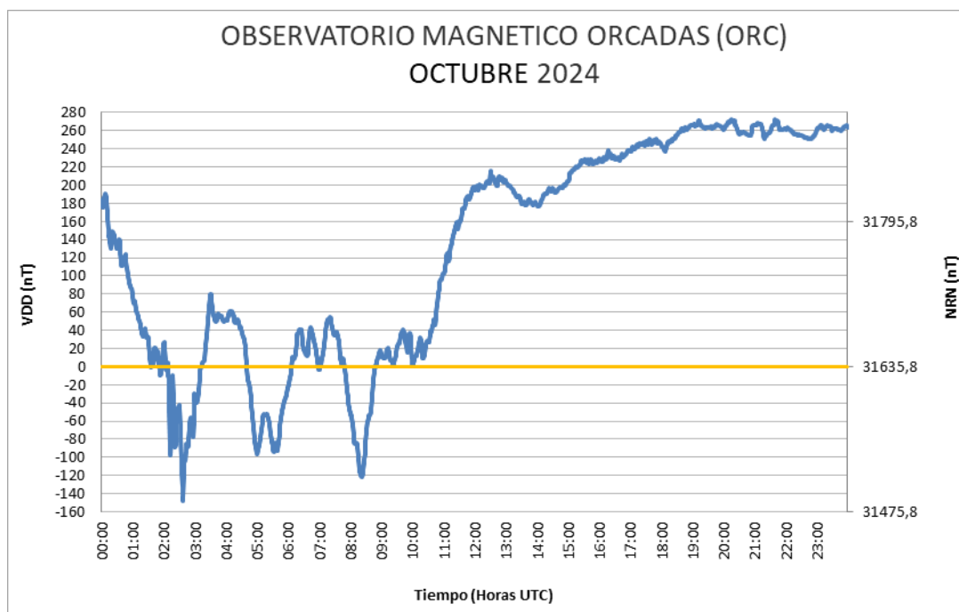
Figura 9: Variación Diaria Perturbada del mes de octubre
