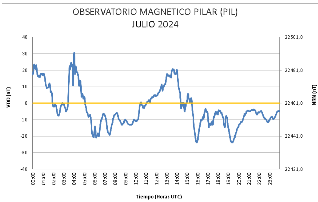
Figura 9: Variación Diaria Perturbada del mes de julio
