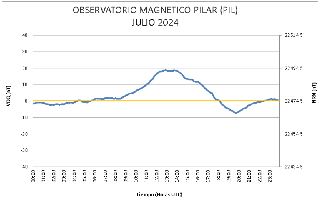
Figura 8: Variación Diaria Calma del mes de julio
