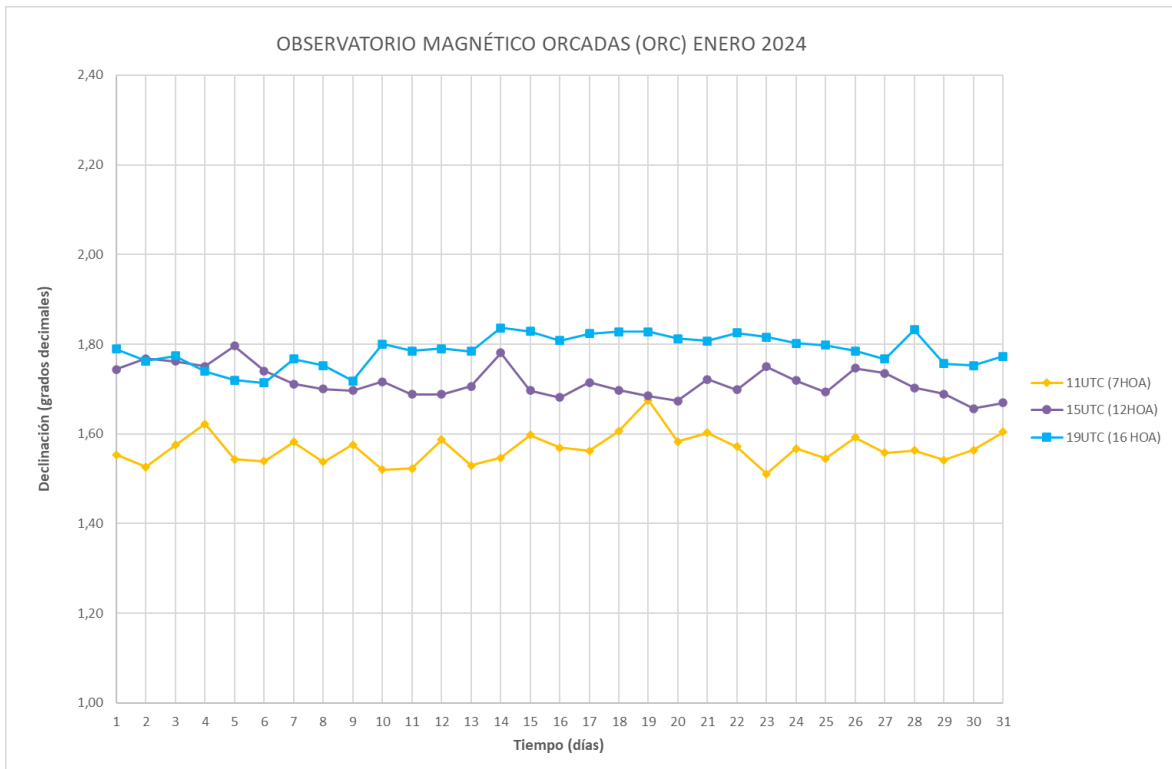
Figura 5: Declinación magnética en función del tiempo
