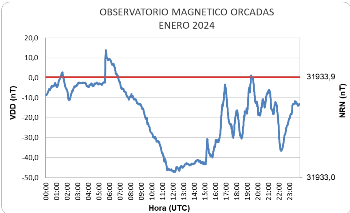
Figura 9: Variación Diaria Perturbada del mes de enero
