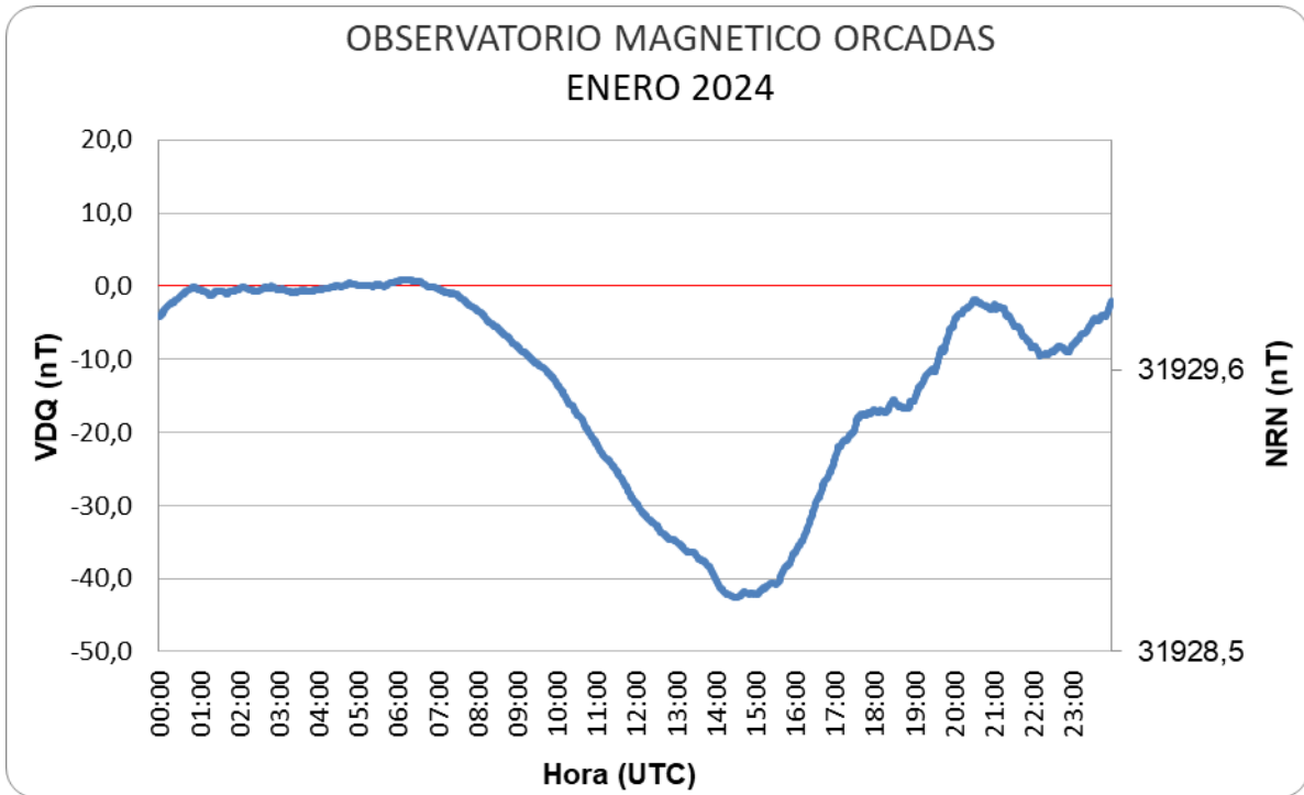
Figura 8: Variación Diaria Calma del mes de enero
