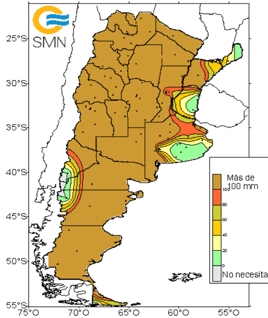
Agua necesaria para comenzar a tener Excesos en los próximos 10 días a partir del 20 de julio de 2023
