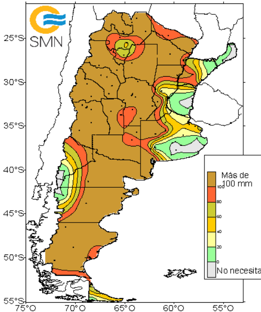
Agua necesaria para tener Buenas Condiciones en los próximos 10 días a partir del 20 de julio de 2023
