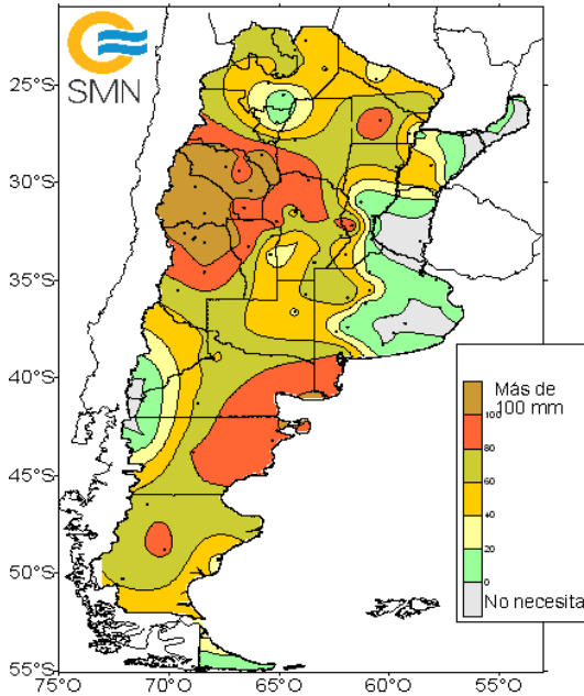
Agua necesaria para no estar en Sequia en los próximos 10 días a partir del 20 de julio de 2023
