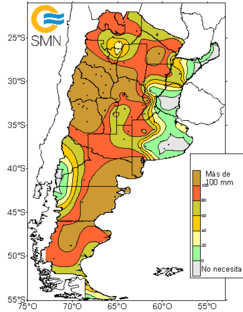
Agua necesaria para no estar en Comienzo de Sequia en los próximos 10 días a partir del 20 de julio de 2023
