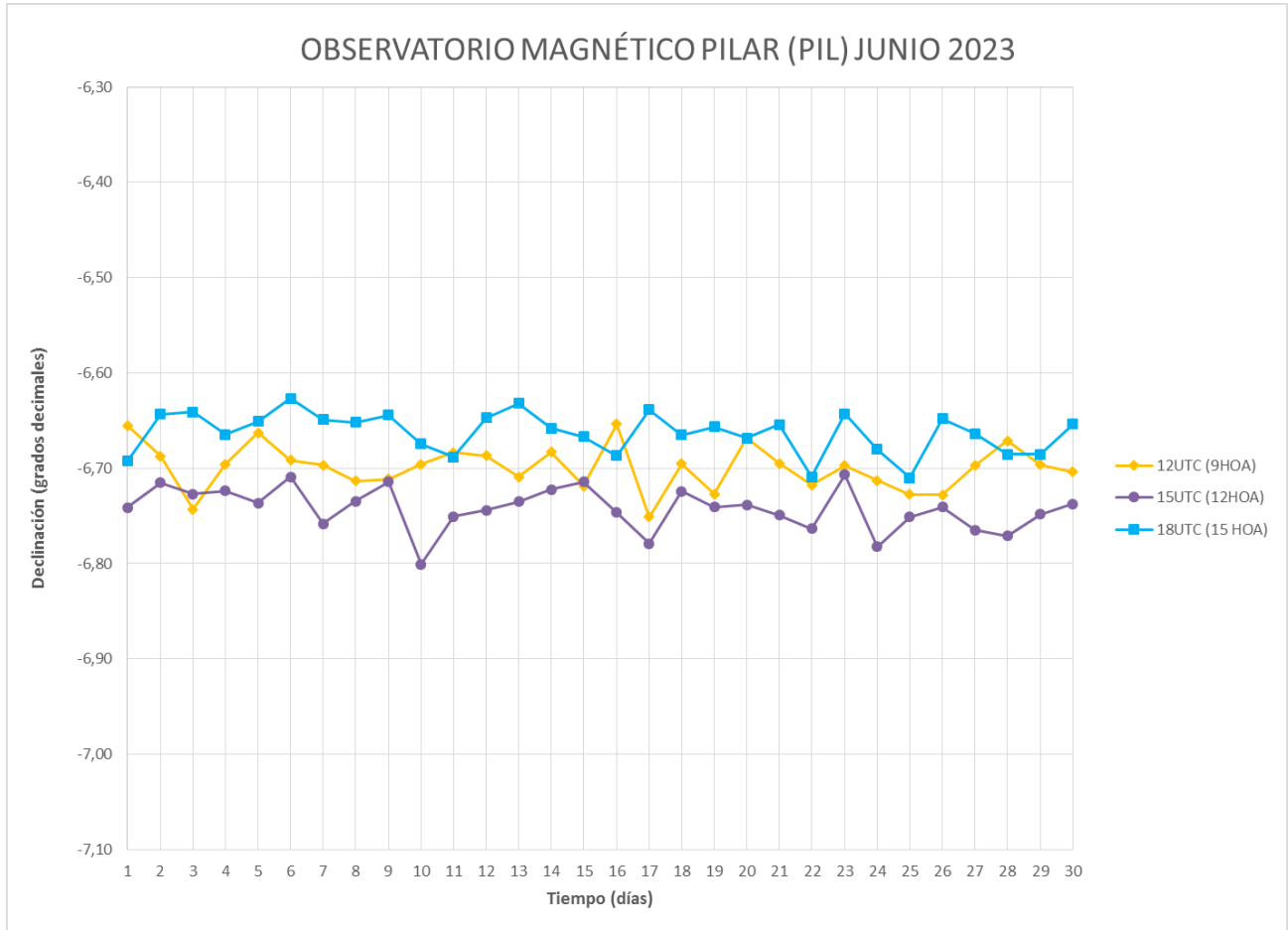
Figura 5: Declinación magnética en función del tiempo
