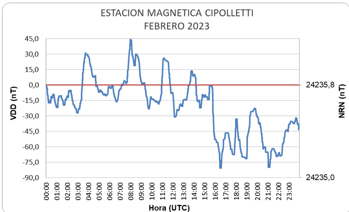
Figura 8: Variación Diaria Perturbada del mes de febrero
