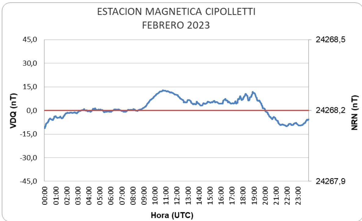
Figura 7: Variación Diaria Calma del mes de febrero
