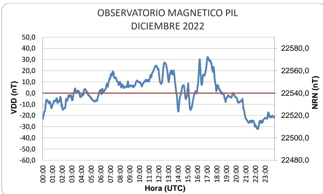
Figura 9: Variación Diaria Perturbada del mes de diciembre
