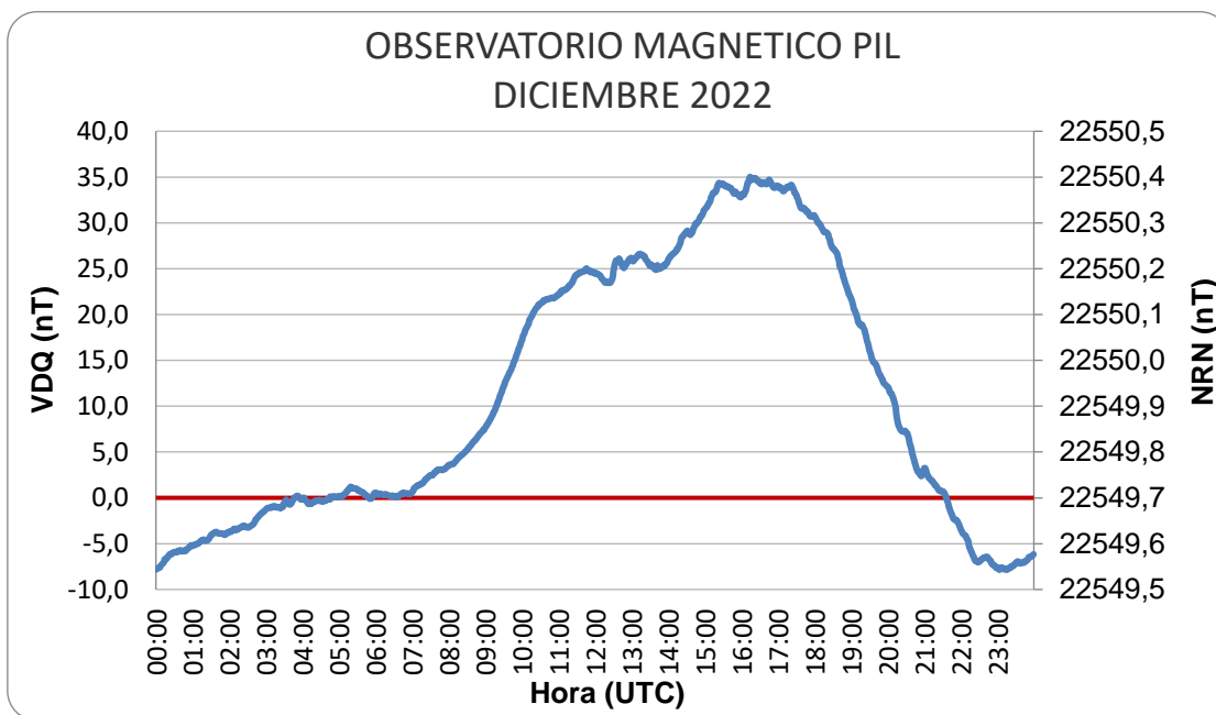
Figura 8: Variación Diaria Calma del mes de diciembre
