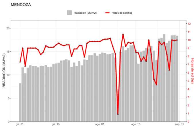
Figura 21. Irradiación solar global diaria y horas de sol obtenidas en Mendoza.
