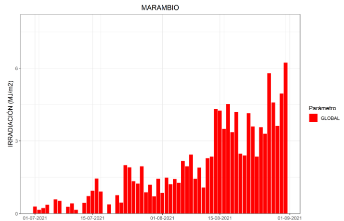
Figura 5. Irradiación solar global diaria disponible para Marambio durante el bimestre considerado
