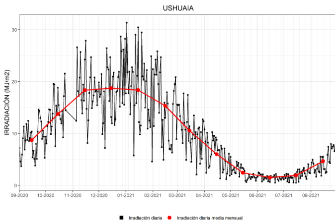
Figura 9. Irradiación solar global diaria y promedios mensuales de los últimos 12 meses en Ushuaia.
