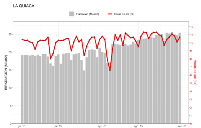
Figura 18. Irradiación solar global diaria y horas de sol obtenidas en La Quiaca.
