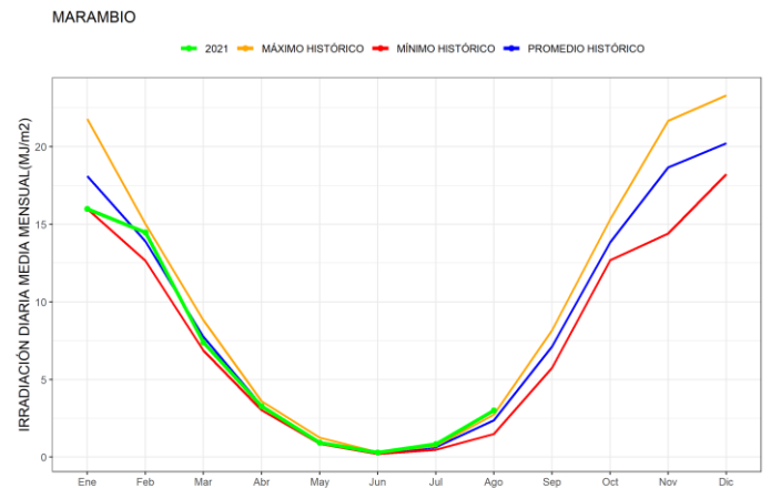
Figura 15. Promedios mensuales de irradiación solar global diaria junto con los valores históricos disponibles de Marambio
