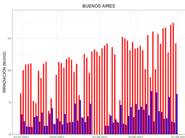
Figura 2. Irradiación solar global y difusa diaria disponibles para Buenos Aires durante el bimestre considerado
