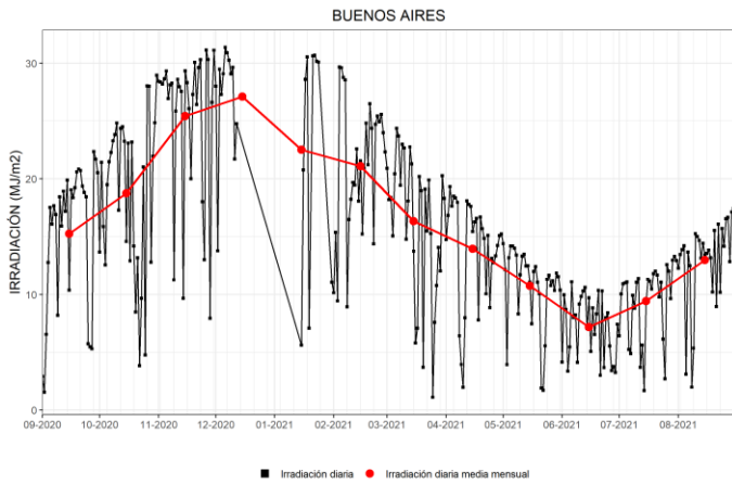
Figura 7. Irradiación solar global diaria y promedios mensuales de los últimos 12 meses en Buenos Aires.
