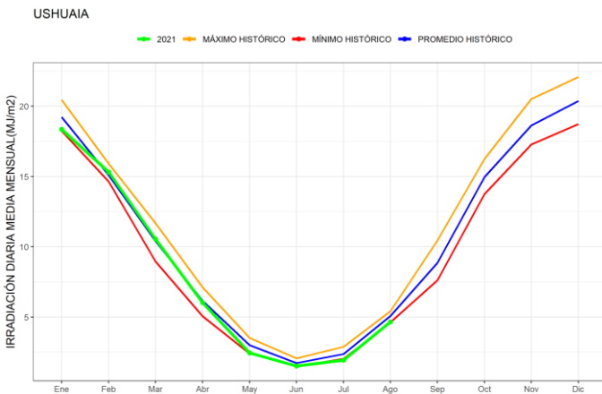
Figura 14. Promedios mensuales de irradiación solar global diaria junto con los valores históricos disponibles de Ushuaia
