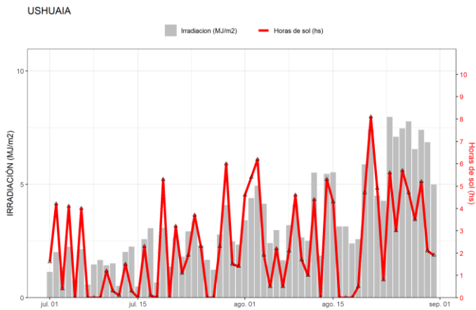
Figura 19. Irradiación solar global diaria y horas de sol obtenidas en Ushuaia.
