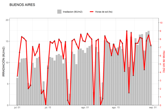
Figura 17. Irradiación solar global diaria y horas de sol obtenidas en Buenos Aires.
