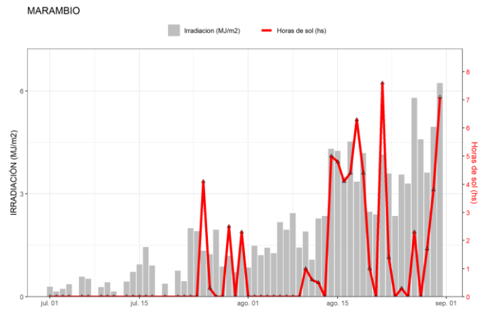
Figura 20. Irradiación solar global diaria y horas de sol obtenidas en Marambio.
