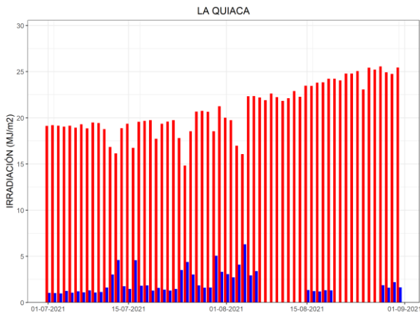
Figura 4. Irradiación solar global y difusa diaria disponibles para La Quiaca durante el bimestre considerado
