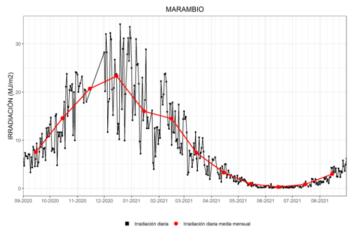
Figura 10. Irradiación solar global diaria y promedios mensuales de los últimos 12 meses en Marambio.
