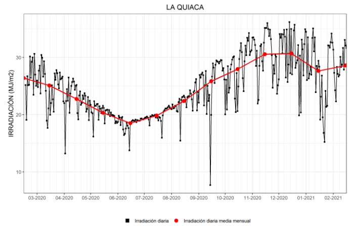
Figura 9. Irradiación solar global diaria y promedios mensuales de los últimos 12 meses en La Quiaca.
