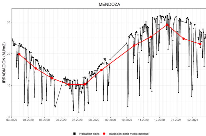
Figura 10. Irradiación solar global diaria y promedios mensuales de los últimos 12 meses en Mendoza.
