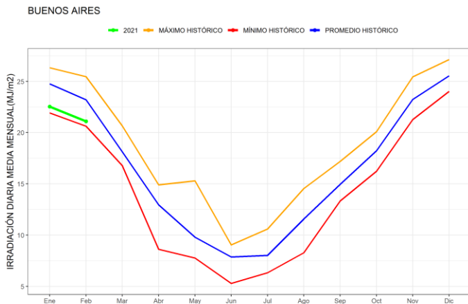
Figura 14. Promedios mensuales de irradiación solar global diaria junto con los valores históricos disponibles de Buenos Aires
