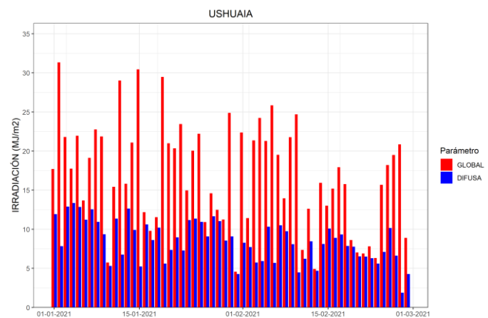
Figura 3. Irradiación solar global y difusa diaria disponibles para Ushuaia durante el bimestre considerado
