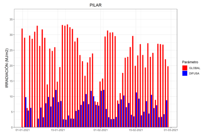
Figura 5. Irradiación solar global y difusa diaria disponibles para Pilar durante el bimestre considerado
