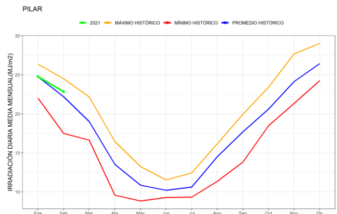
Figura 15. Promedios mensuales de irradiación solar global diaria junto con los valores históricos disponibles de Pilar
