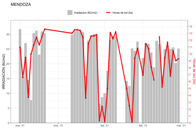
Figura 24. Irradiación solar global diaria y horas de sol obtenidas en Mendoza.
