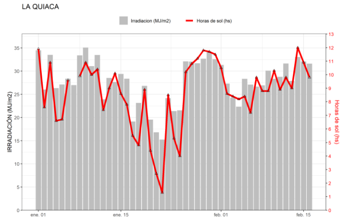
Figura 23. Irradiación solar global diaria y horas de sol obtenidas en La Quiaca.
