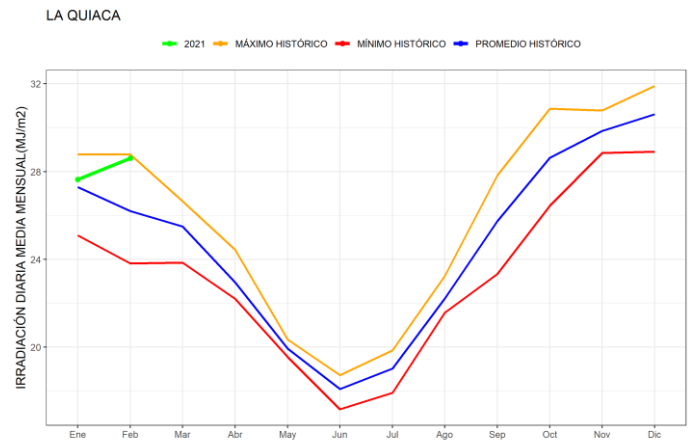
Figura 19. Promedios mensuales de irradiación solar global diaria junto con los valores históricos disponibles de Mendoza
