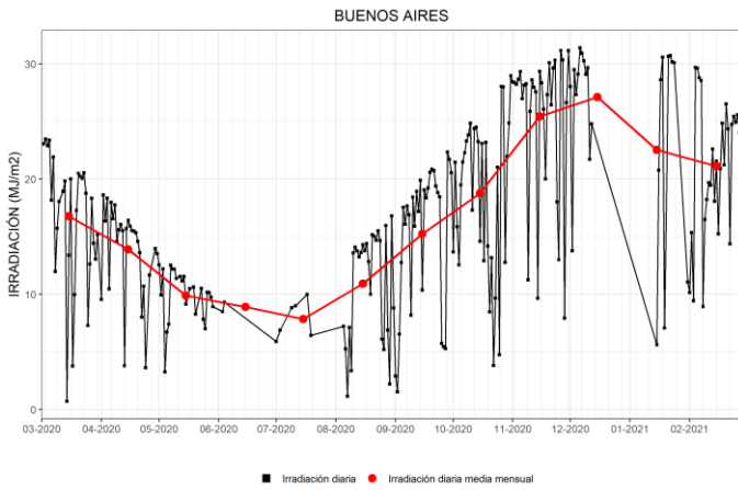
Figura 8. Irradiación solar global diaria y promedios mensuales de los últimos 12 meses en Buenos Aires.
