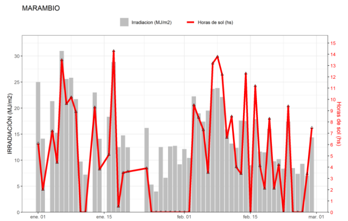
Figura 25. Irradiación solar global diaria y horas de sol obtenidas en Marambio.
