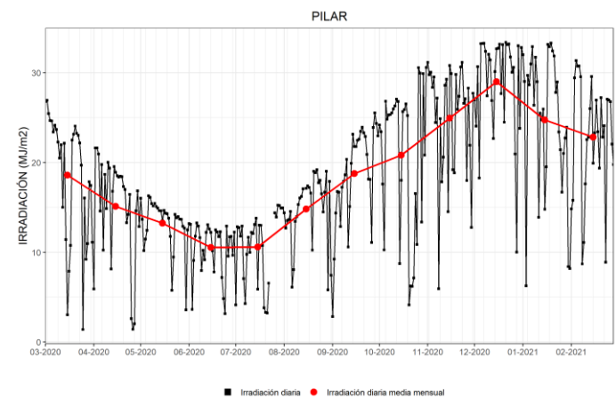
Figura 13. Irradiación solar global diaria y promedios mensuales de los últimos 12 meses en Pilar.
