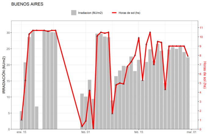
Figura 22. Irradiación solar global diaria y horas de sol obtenidas en Buenos Aires.
