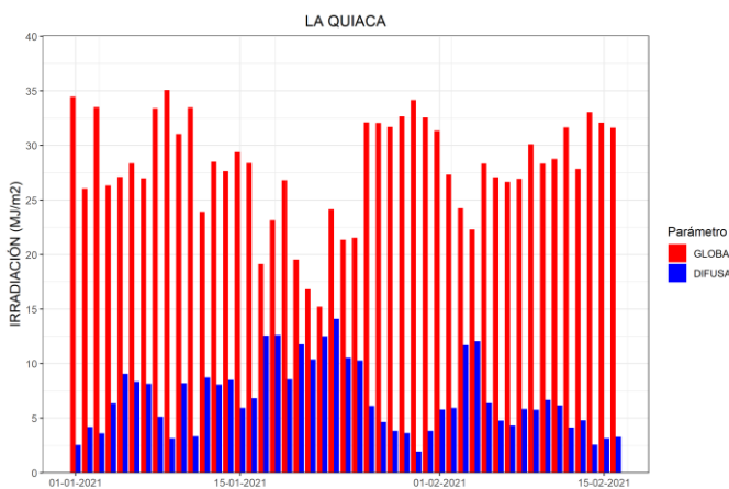
Figura 2. Irradiación solar global y difusa diaria disponibles para La Quiaca durante el bimestre considerado
