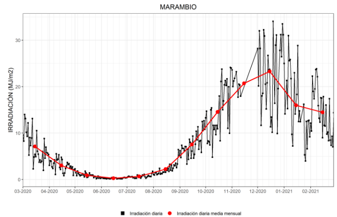
Figura 11. Irradiación solar global diaria y promedios mensuales de los últimos 12 meses en Marambio.
