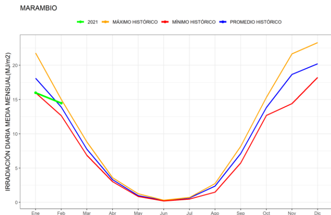
Figura 16. Promedios mensuales de irradiación solar global diaria junto con los valores históricos disponibles de Marambio
