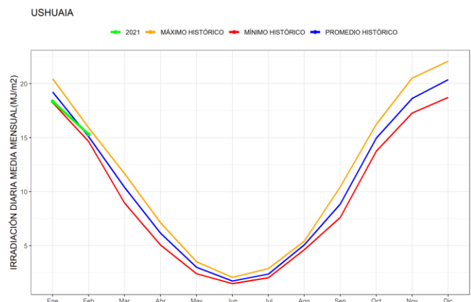
Figura 17. Promedios mensuales de irradiación solar global diaria junto con los valores históricos disponibles de Ushuaia
