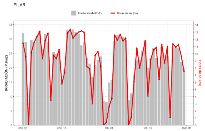
Figura 21. Irradiación solar global diaria y horas de sol obtenidas en Pilar.
