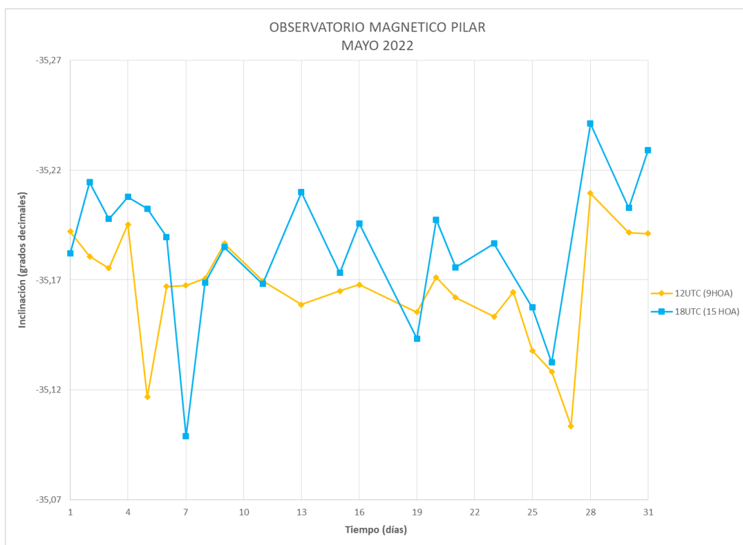
Figura 6: Inclínación magnética en función del tiempo
