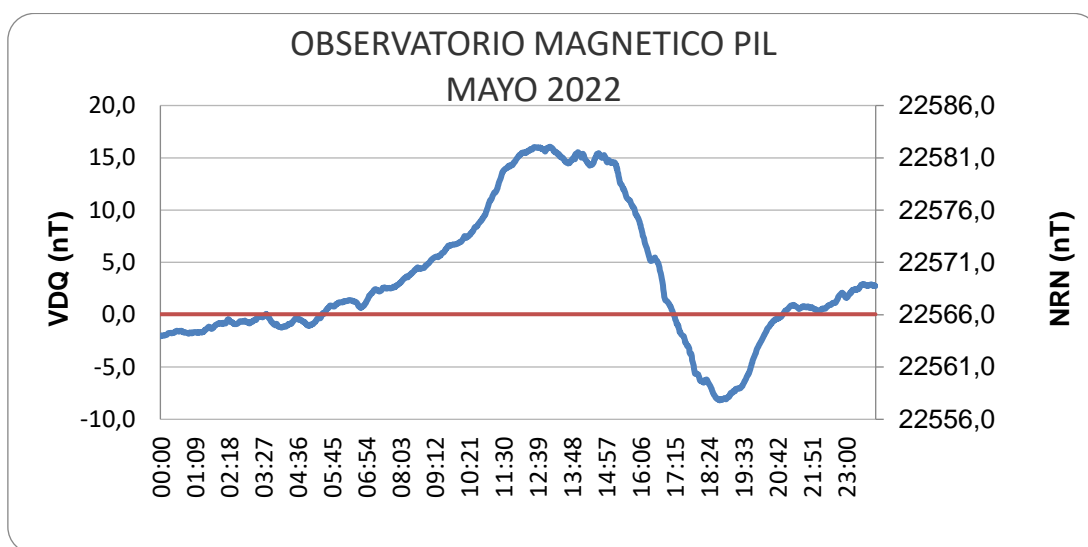
Figura 8: Variación Diaria Calma del mes de mayo
