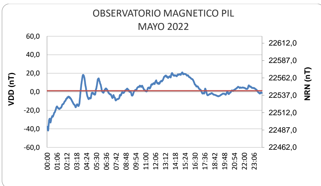
Figura 9: Variación Diaria Perturbada del mes de mayo
