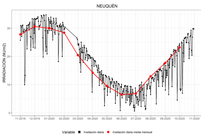
Figura 18. Irradiación solar global diaria y promedios mensuales de los últimos 12 meses en Neuquén.
