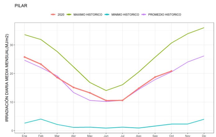
Figura 24. Promedios mensuales de irradiación solar global diaria junto con los valores históricos disponibles de Pilar
