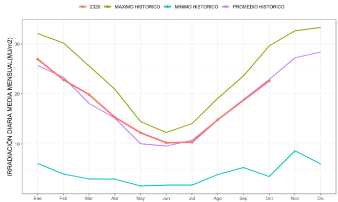
Figura 28. Promedios mensuales de irradiación solar global diaria junto con los valores históricos disponibles de Mendoza
