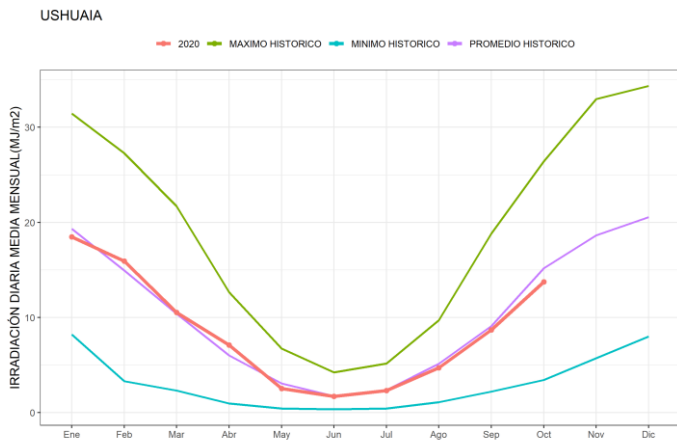
Figura 21. Promedios mensuales de irradiación solar global diaria junto con los valores históricos disponibles de Ushuaia
