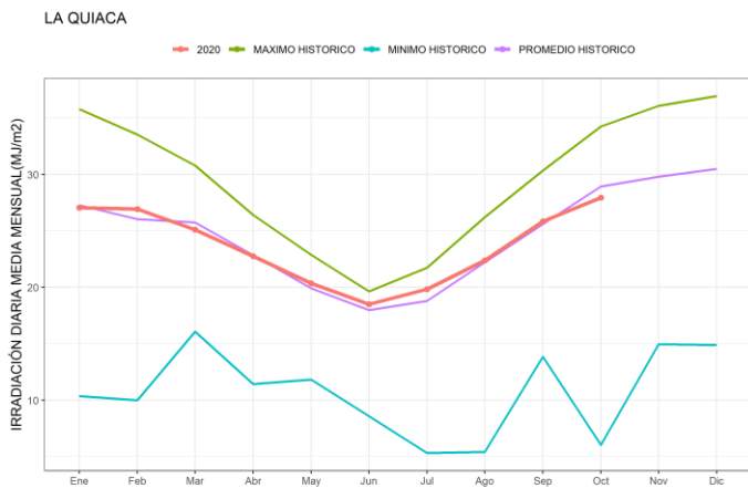
Figura 23. Promedios mensuales de irradiación solar global diaria junto con los valores históricos disponibles de La Quiaca
