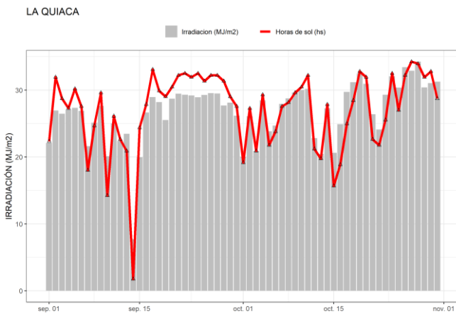
Figura 32. Irradiación solar global diaria y horas de sol obtenidas en La Quiaca.
