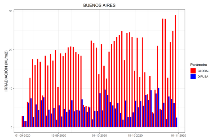
Figura 4. Irradiación solar global y difusa diaria disponible para Buenos Aires durante el bimestre considerado
