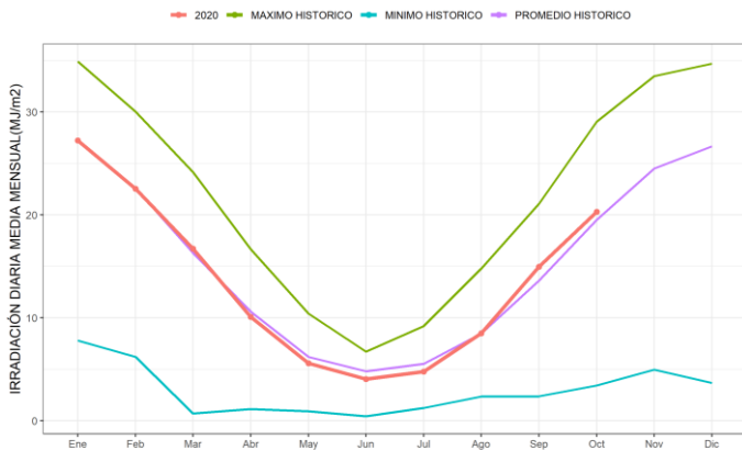
Figura 29. Promedios mensuales de irradiación solar global diaria junto con los valores históricos disponibles de Com. Rivadavia
