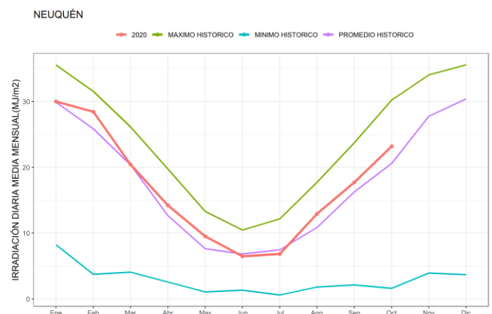
Figura 26. Promedios mensuales de irradiación solar global diaria junto con los valores históricos disponibles de Neuquén
