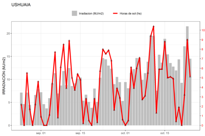
Figura 30. Irradiación solar global diaria y horas de sol obtenidas en Ushuaia.
