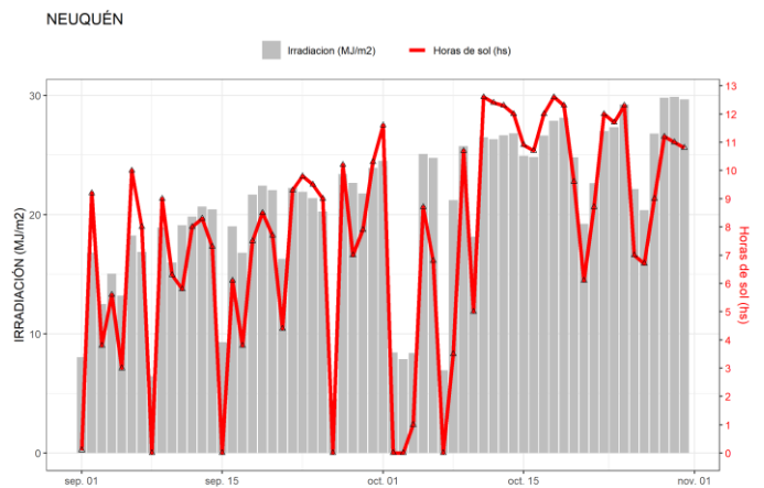
Figura 35. Irradiación solar global diaria y horas de sol obtenidas en Neuquén.
