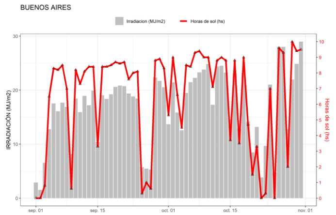
Figura 31. Irradiación solar global diaria y horas de sol obtenidas en Buenos Aires.
