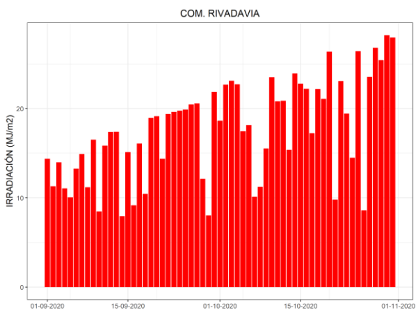
Figura 9. Irradiación solar global diaria disponible para Com. Rivadavia durante el bimestre considerado
