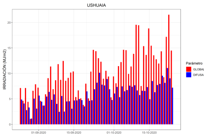
Figura 3. Irradiación solar global y difusa diaria disponible para Ushuaia durante el bimestre considerado
