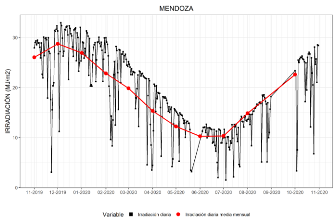
Figura 17. Irradiación solar global diaria y promedios mensuales de los últimos 12 meses en Mendoza.
