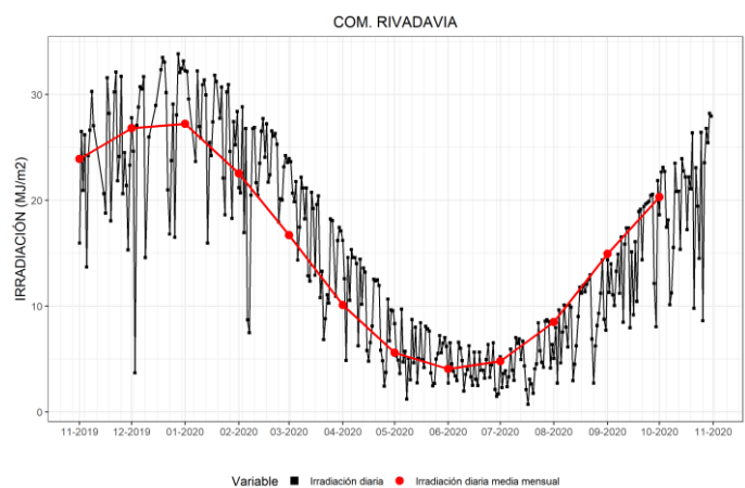
Figura 19. Irradiación solar global diaria y promedios mensuales de los últimos 12 meses en Com. Rivadavia.
