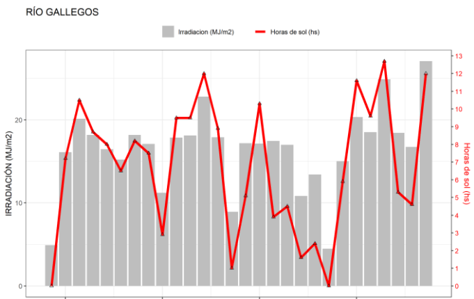
Figura 34. Irradiación solar global diaria y horas de sol obtenidas en Río Gallegos.
