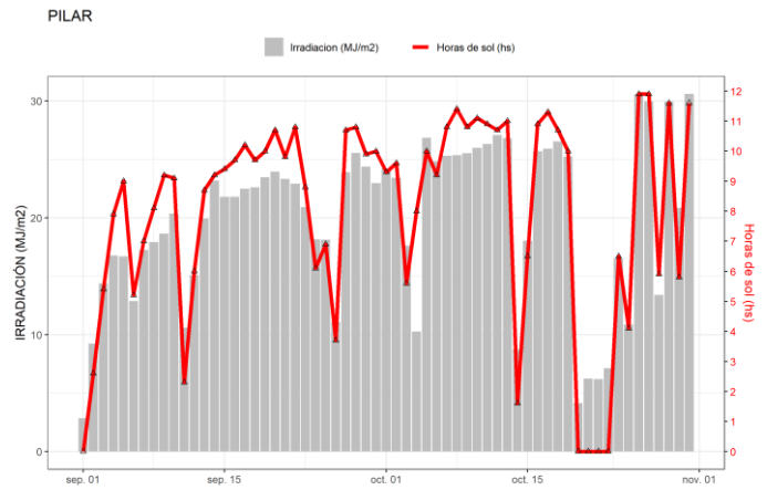
Figura 33. Irradiación solar global diaria y horas de sol obtenidas en Pilar.
