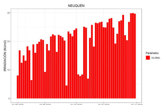
Figura 10. Irradiación solar global diaria disponible para Neuquén durante el bimestre considerado
