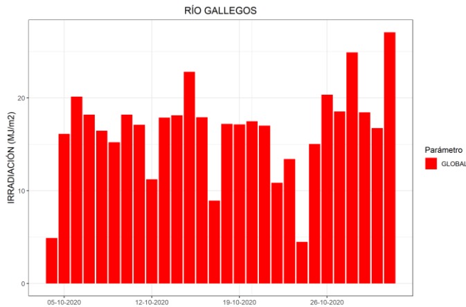
Figura 11. Irradiación solar global diaria disponible para Rio Gallegos durante el bimestre considerado
