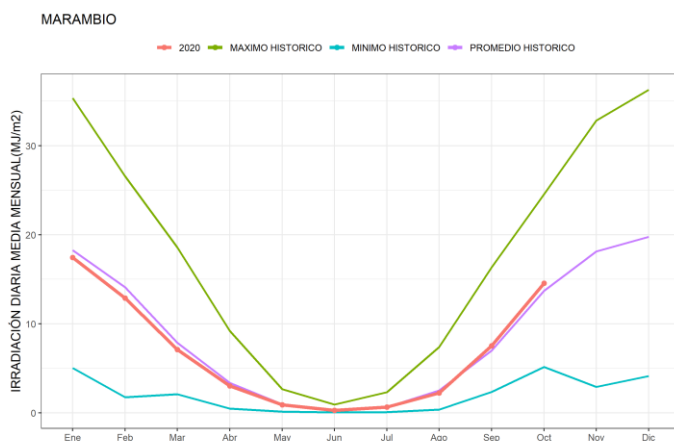
Figura 25. Promedios mensuales de irradiación solar global diaria junto con los valores históricos disponibles de Marambio
