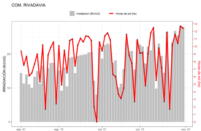
Figura 38. Irradiación solar global diaria y horas de sol obtenidas en Com. Rivadavia.
