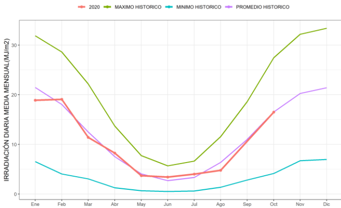
Figura 27. Promedios mensuales de irradiación solar global diaria junto con los valores históricos disponibles de Río Gallegos
