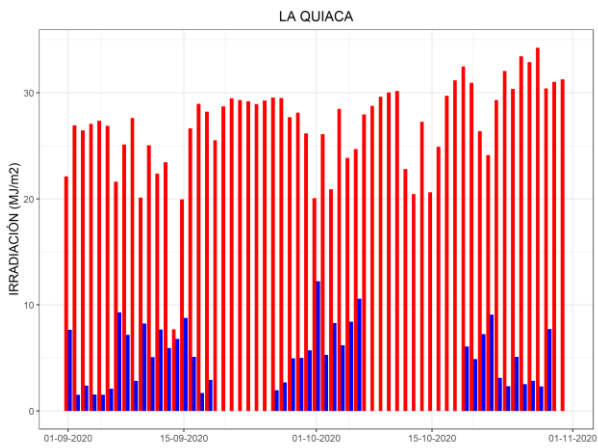
Figura 5. Irradiación solar global y difusa diaria disponible para La Quiaca durante el bimestre considerado
