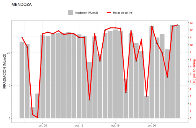
Figura 36. Irradiación solar global diaria y horas de sol obtenidas en Mendoza.
