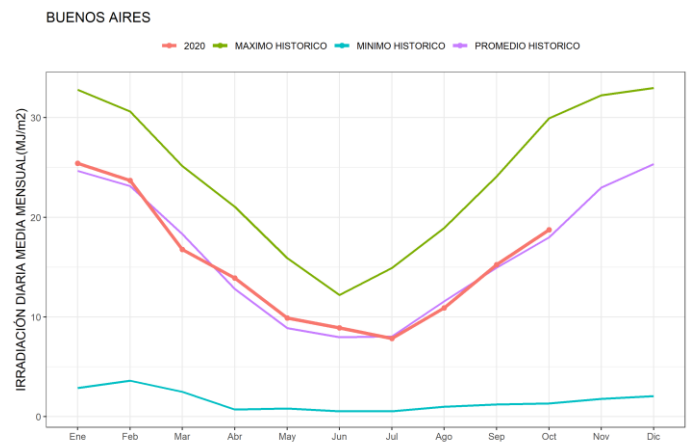
Figura 22. Promedios mensuales de irradiación solar global diaria junto con los valores históricos disponibles de Buenos Aires
