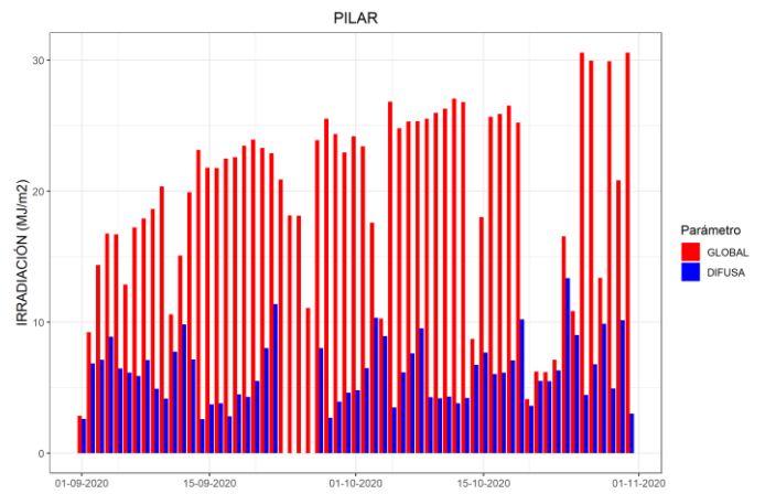
Figura 6. Irradiación solar global y difusa diaria disponible para Pilar durante el bimestre considerado
