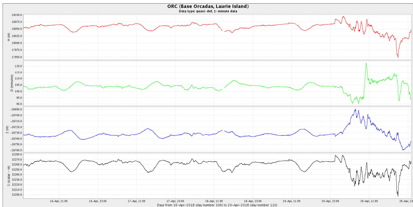
Figura 4b: Componentes del campo magnético del 11 al 20 de abril. En rojo se ve la componente horizontal (H) y en azul la vertical (Z), ambas en nT. En verde se presenta la declinación del campo magnético (D) en minutos y en negro la intensidad del campo magnético en nT.
