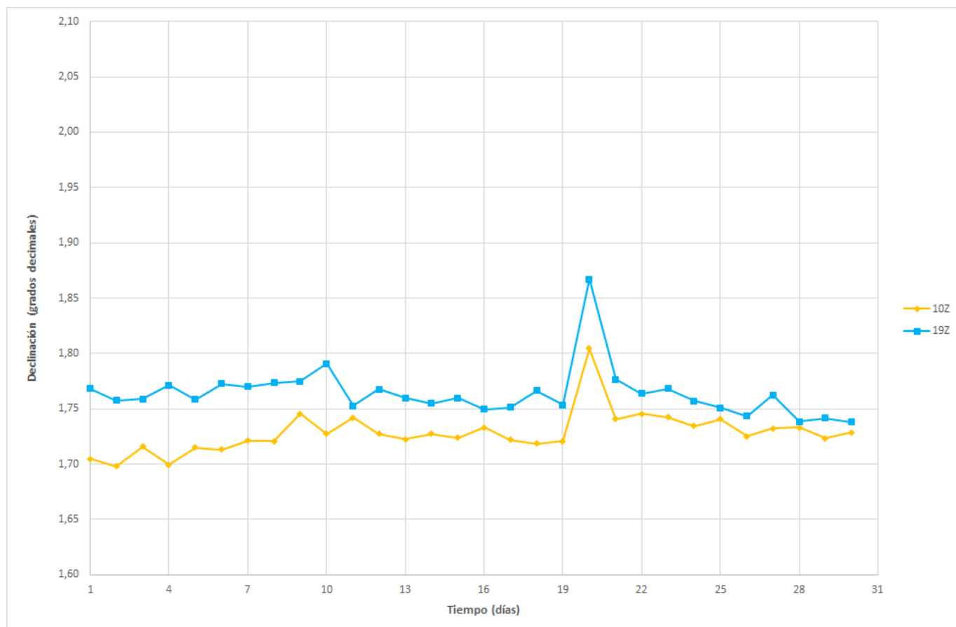
Figura 5: Declinación magnética en función del tiempo
