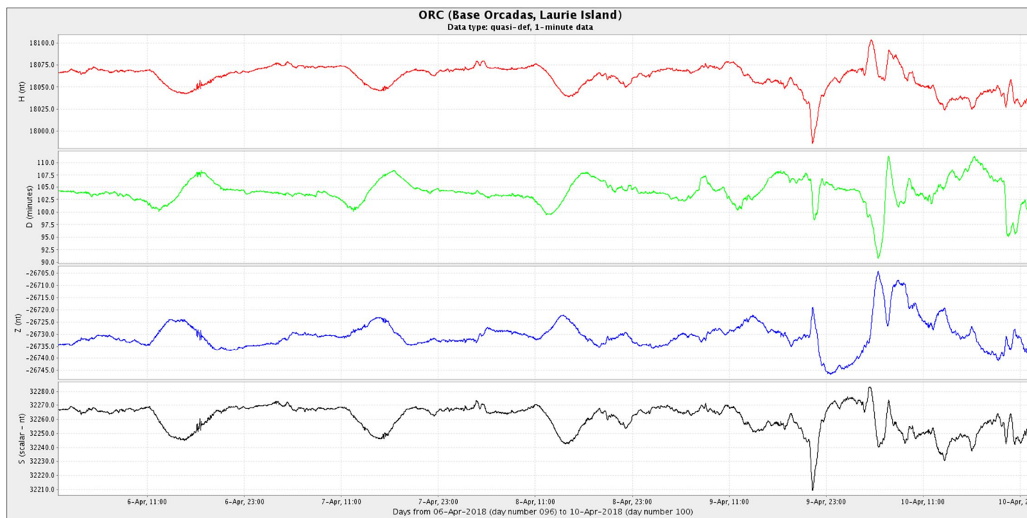
Figura 4a: Componentes del campo magnético del 1 al 10 de abril. En rojo se ve la componente horizontal (H) y en azul la vertical (Z), ambas en nT. En verde se presenta la declinación del campo magnético (D) en minutos y en negro la intensidad del campo magnético en nT
