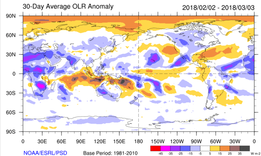
Figura 6 – Anomalías de radiación de onda larga saliente (OLR) del 2 de febrero al 3 de marzo de 2018 - Fuente: NOAA-CIRES/CDC
