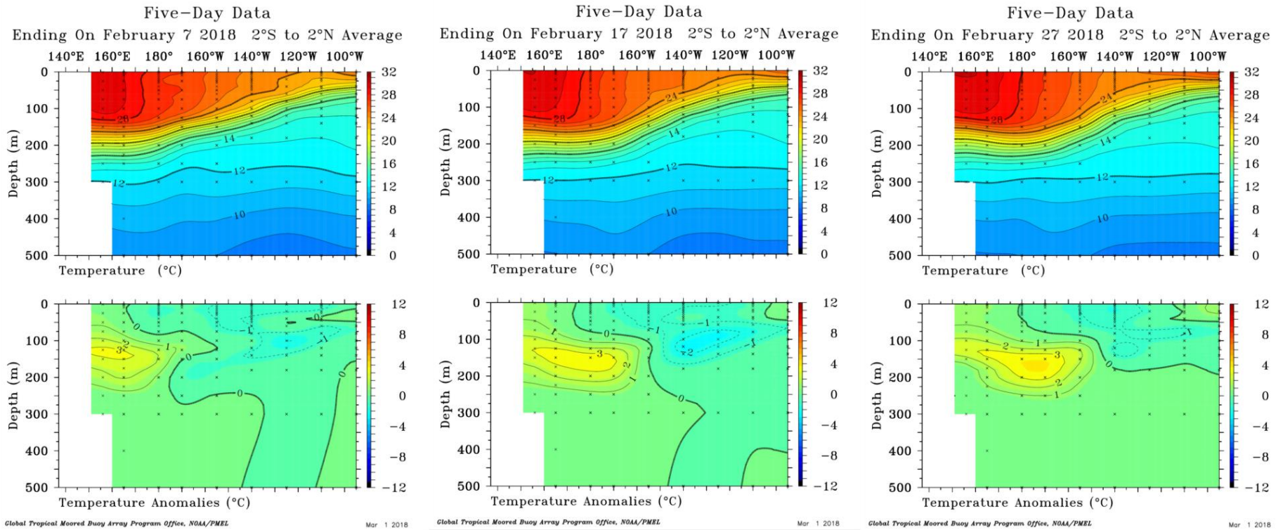
Figura 4 – Corte profundidad vs. Longitud de la TSM y sus anomalías, en el Pacífico ecuatorial, correspondientes al 03-07 de febrero (izquierda), al 13-17 de febrero (centro) y al 23 -27 de febrero de 2018 (derecha). Fuente: PMEL - NOA.
