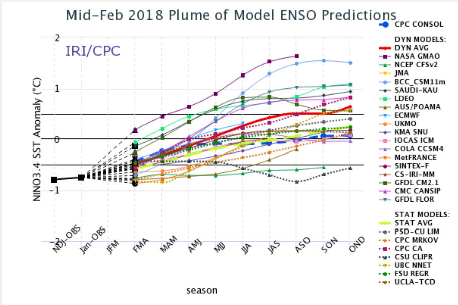
Figura 8 – Pronóstico de anomalías de TSM en la región Niño 3.4. Fuente: IRI.
