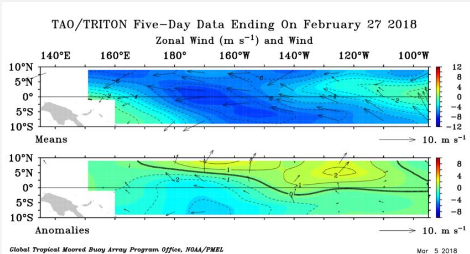
Figura 5 – Viento zonal y anomalías del 23 al 27 de febrero de 2018 - Fuente: PMEL - NOAA.
