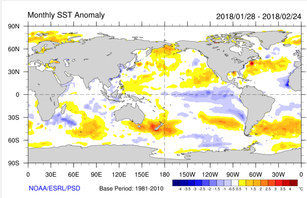
Figura 1: Anomalías de la temperatura superficial del mar en febrero de 2018. Período de referencia 1981-2010 - Fuente: NOAA-CIRES/CDC
