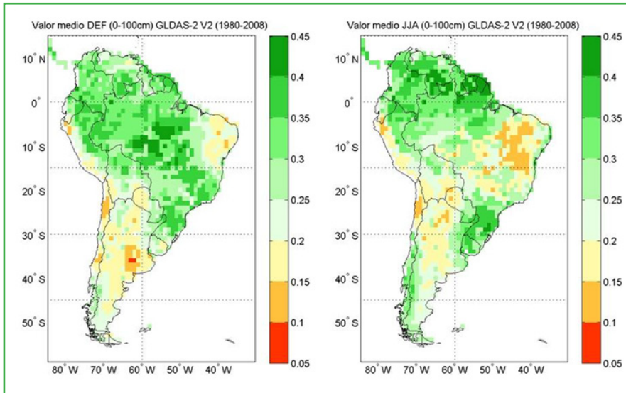
Campos medios de humedad del suelo ( \text{m}^3/\text{m}^3 , espesor 0-100cm) para verano (DEF) e invierno (JJA) según GLDAS-2.0. Figura tomada de Spennemann (2015).
