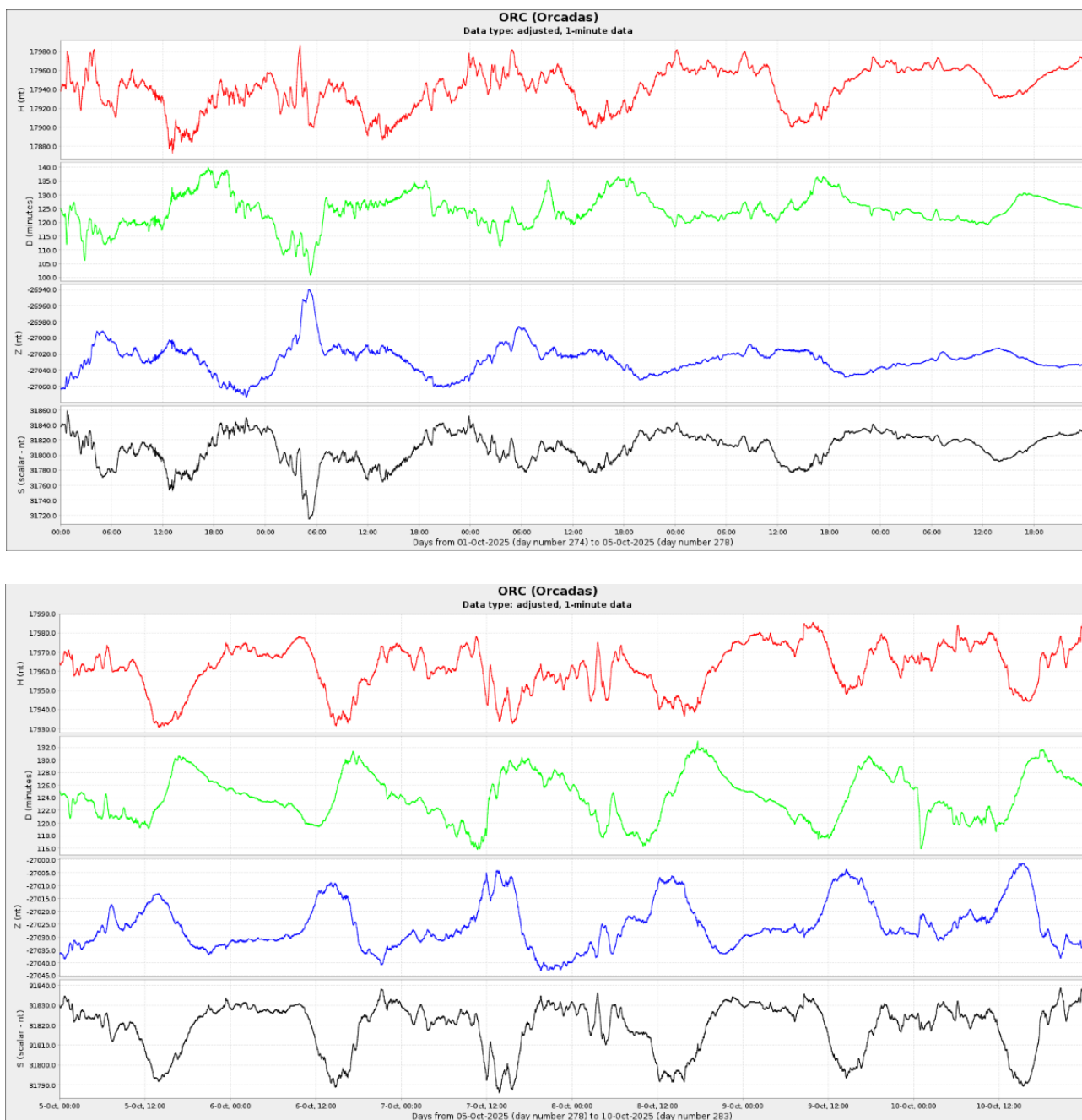
Figura 4a: Componentes del campo magnético del 1 al 10 de octubre. En rojo se ve la componente horizontal (H) y en azul la vertical (Z), ambas en nT. En verde se presenta la declinación del campo magnético (D) en minutos y en negro la intensidad del campo magnético en nT
