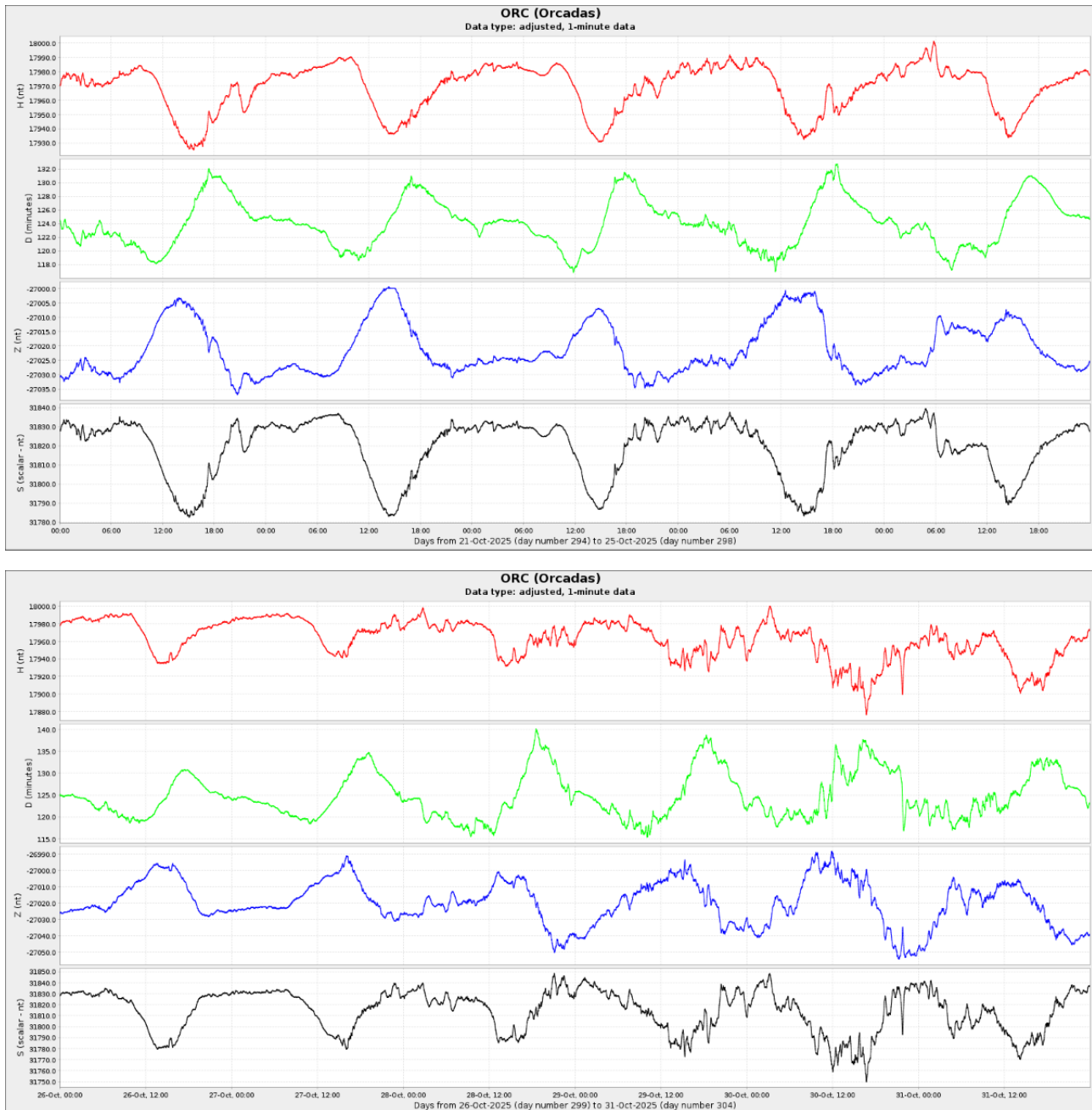
Figura 4c: Componentes del campo magnético del 21 al 31 de octubre. En rojo se ve la componente horizontal (H) y en azul la vertical (Z), ambas en nT. En verde se presenta la declinación del campo magnético (D) en minutos y en negro la intensidad del campo magnético en Nt, dejando la aclaración la ausencia de datos de la intensidad del campo magnético debido a mantenimiento del sistema indigo.
