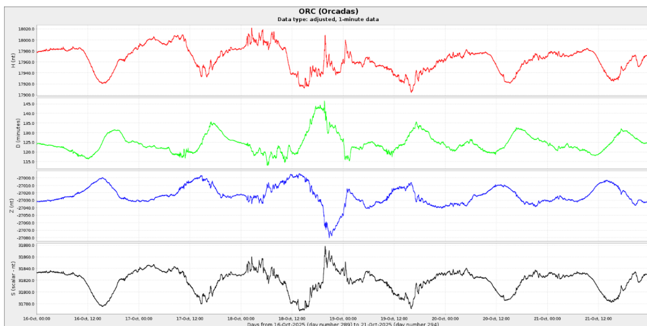
Figura 4b Componentes del campo magnético del 11 al 21 de octubre. En rojo se ve la componente horizontal (H) y en azul la vertical (Z), ambas en nT. En verde se presenta la declinación del campo magnético (D) en minutos y en negro la intensidad del campo magnético en nT.
