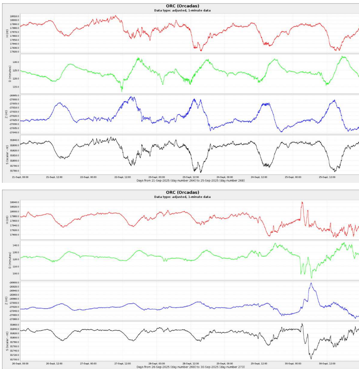
Figura 4c: Componentes del campo magnético del 21 al 30 de septiembre. En rojo se ve la componente horizontal (H) y en azul la vertical (Z), ambas en nT. En verde se presenta la declinación del campo magnético (D) en minutos y en negro la intensidad del campo magnético en Nt, dejando la aclaración la ausencia de datos de la intensidad del campo magnético debido a mantenimiento del sistema indigo.
