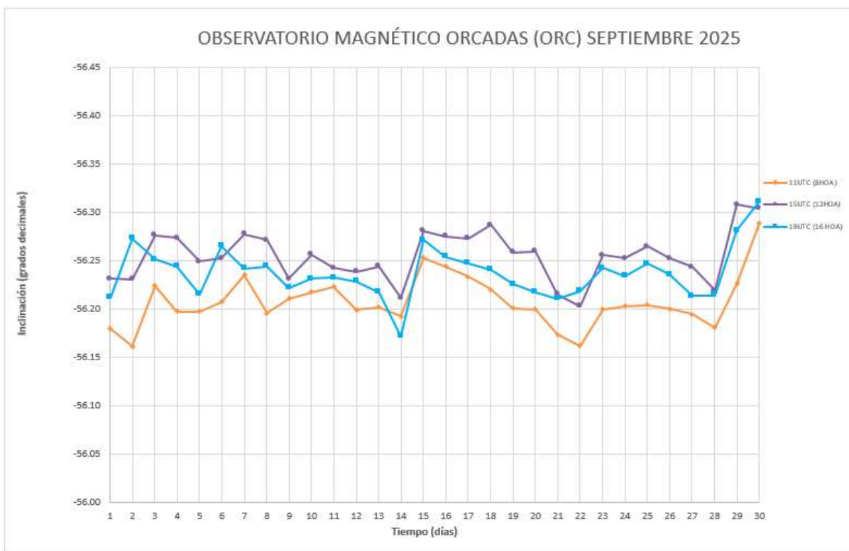
Figura 6: Inclínación magnética en función del tiempo
