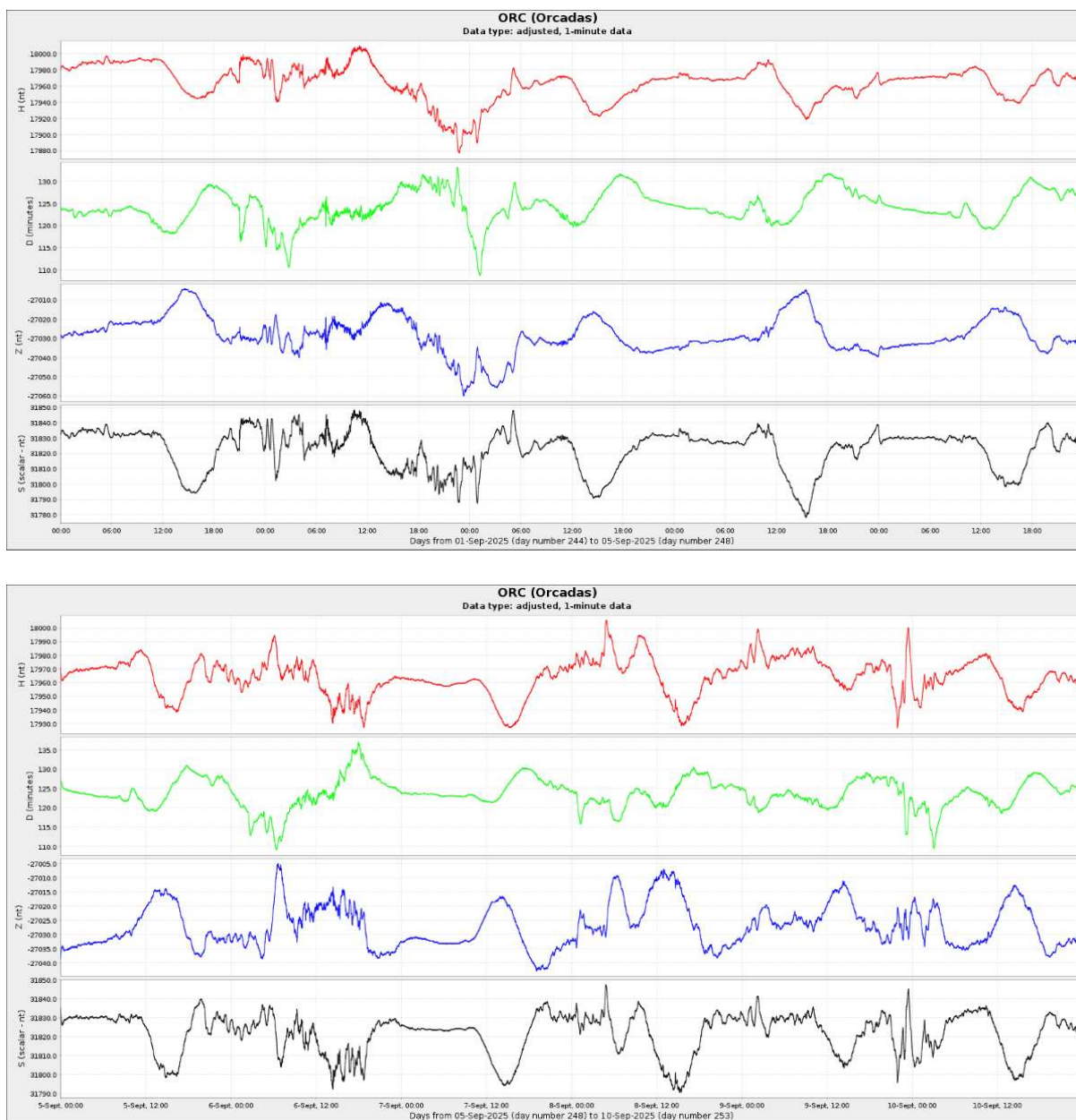
Figura 4a: Componentes del campo magnético del 1 al 10 de septiembre. En rojo se ve la componente horizontal (H) y en azul la vertical (Z), ambas en nT. En verde se presenta la declinación del campo magnético (D) en minutos y en negro la intensidad del campo magnético en nT
