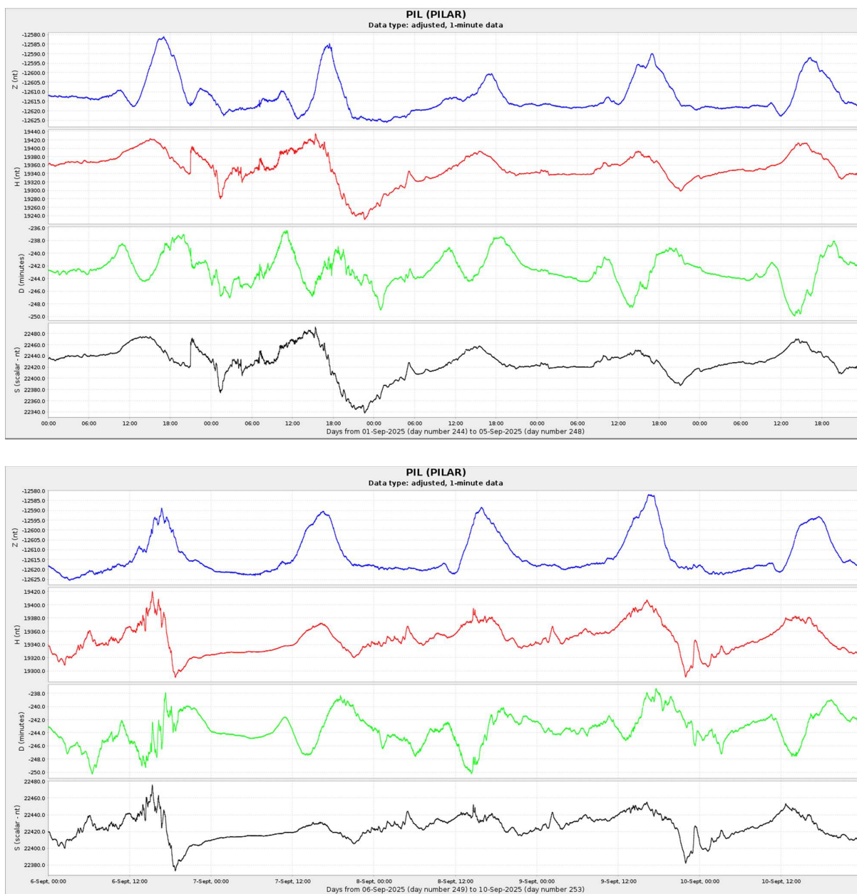
Figura 4a: Componentes del campo magnético del día 1 al 10 de septiembre. En rojo se ve la componente horizontal (H) y en azul la vertical (Z), ambas en nT. En verde se presenta la declinación del campo magnético (D) en minutos y en negro la intensidad del campo magnético en nT.
