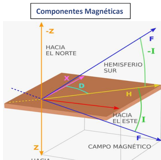
Figura 3: Componentes del campo magnético
