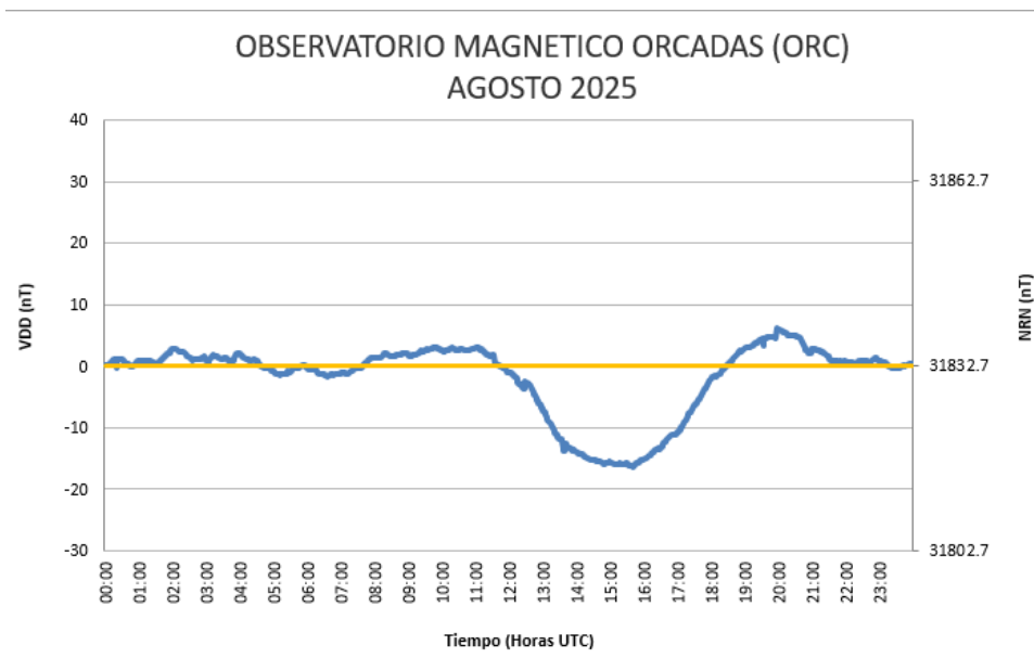
Figura 8: Variación Diaria Calma del mes de agosto
