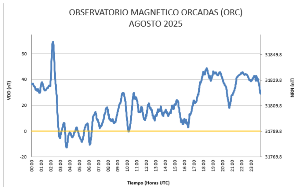
Figura 9: Variación Diaria Perturbada del mes de agosto
