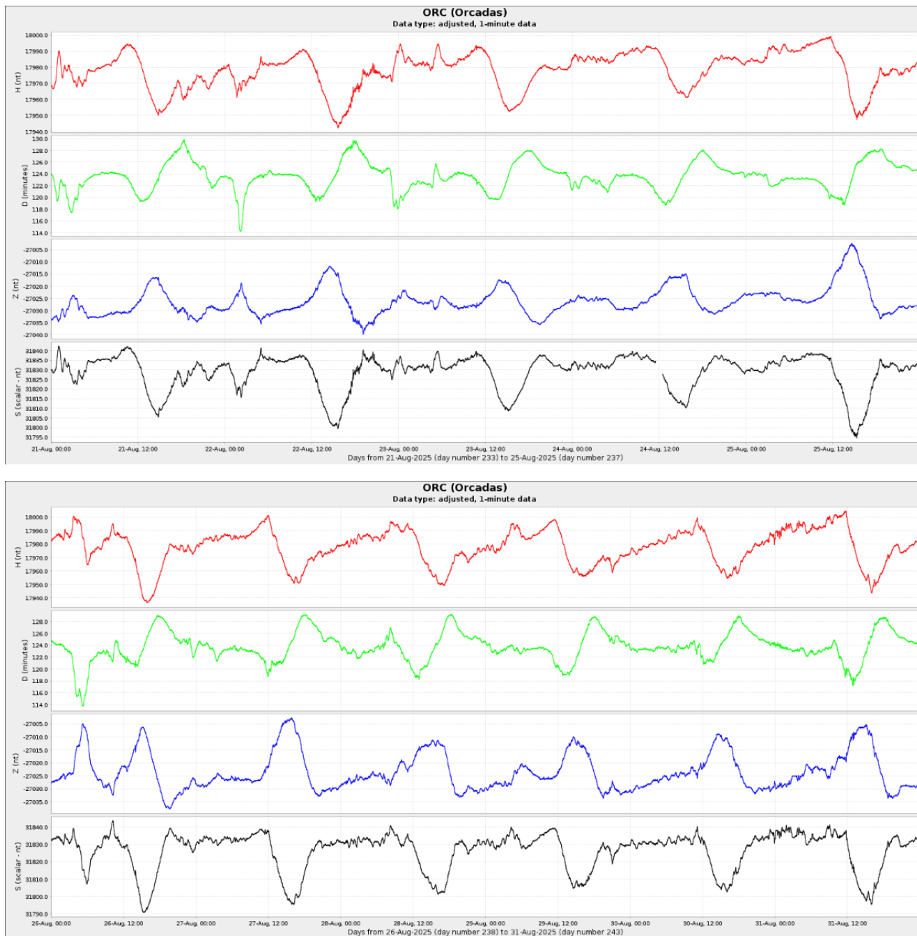
Figura 4c: Componentes del campo magnético del 21 al 31 de agosto. En rojo se ve la componente horizontal ( H ) y en azul la vertical ( Z ), ambas en nT. En verde se presenta la declinación del campo magnético ( D ) en minutos y en negro la intensidad del campo magnético en Nt, dejando la aclaración la ausencia de datos de la intensidad del campo magnético debido a mantenimiento del sistema indigo.
