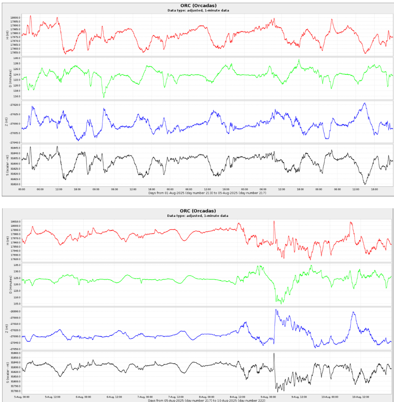
Figura 4a: Componentes del campo magnético del 1 al 10 de agosto. En rojo se ve la componente horizontal (H) y en azul la vertical (Z), ambas en nT. En verde se presenta la declinación del campo magnético (D) en minutos y en negro la intensidad del campo magnético en nT
