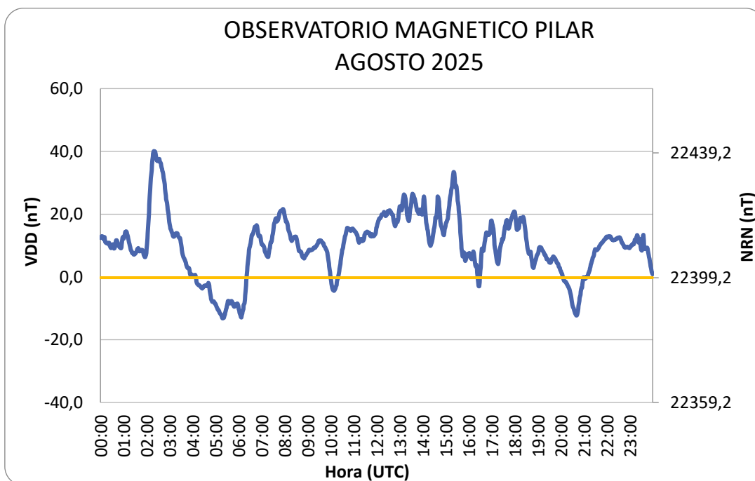
Figura 9: Variación Diaria Perturbada del mes de agosto
