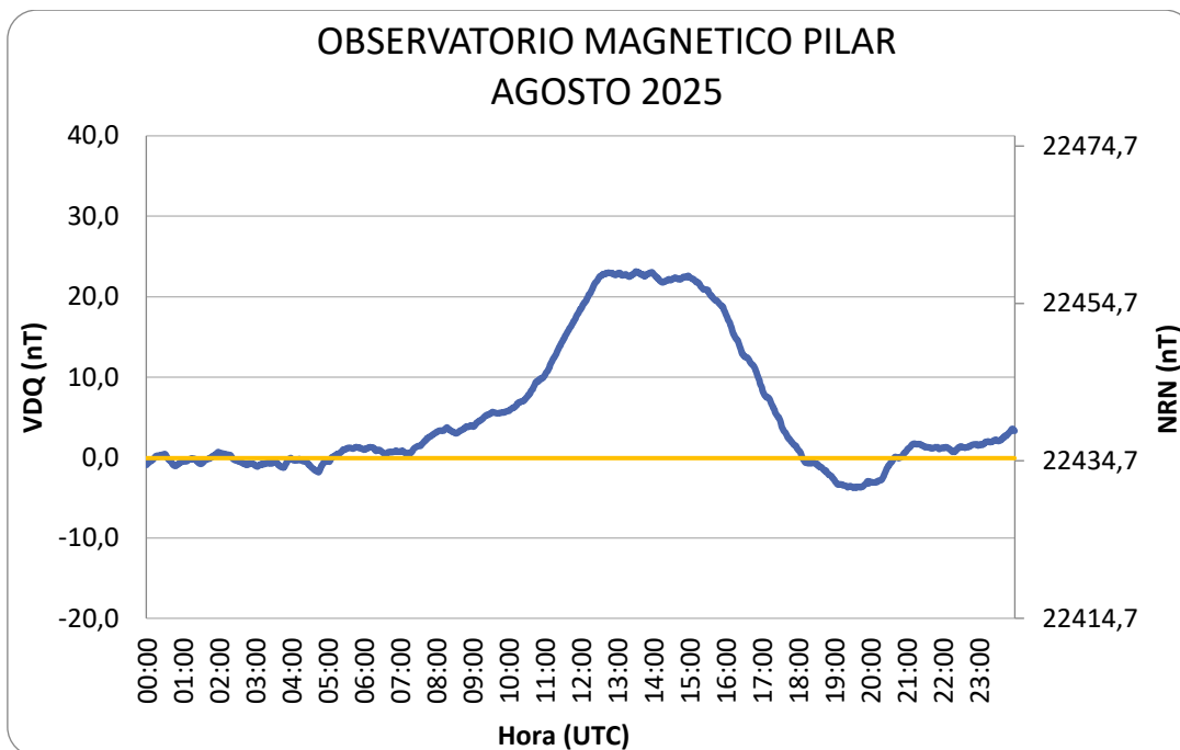
Figura 8: Variación Diaria Calma del mes de agosto
