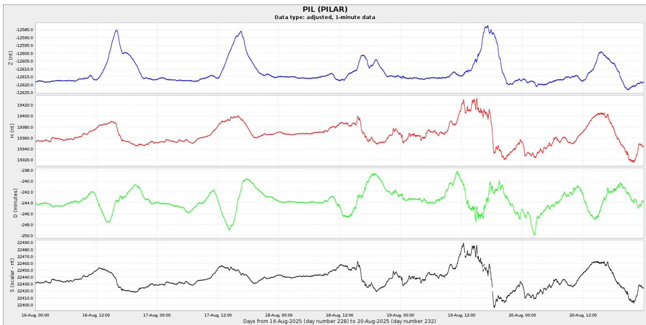
Figura 4b: Componentes del campo magnético del 11 al 20 de agosto. En rojo se ve la componente horizontal (H) y en azul la vertical (Z), ambas en nT. En verde se presenta la declinación del campo magnético (D) en minutos y en negro la intensidad del campo magnético en nT.
