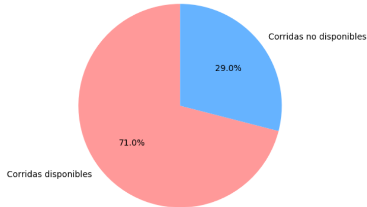
Fig. 6: Proporción de corridas de 12Z del WRF-SMN disponibles en relación con la cantidad total en días donde se cumple el criterio propuesto de tormenta eléctrica
