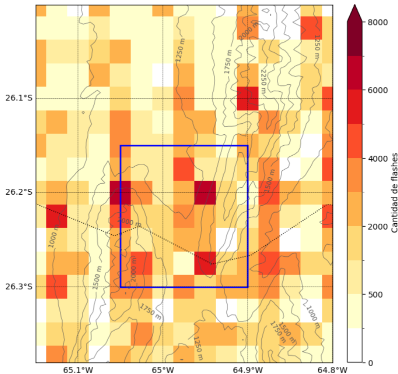
Fig. 9: Distribución espacial de flashes detectados por el sensor GLM del GOES-16, en casos que cumplen con el criterio de detección propuesto en el valle. Los colores representan la cantidad de detecciones en cada cuadrante, con una mayor concentración de eventos en las zonas en tonalidades más oscuras. El recuadro azul indica la región de interés analizada en el estudio.
