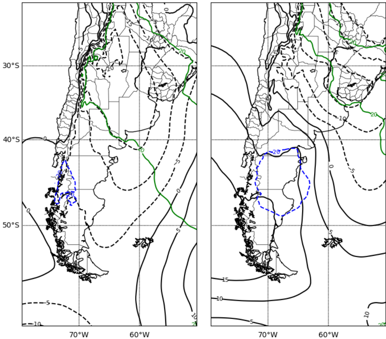
Fig. 12: Anomalías de intensidad de espesores de la capa 1000-500 hPa y de altura geopotencial en 500 hPa. Izquierda: considerando el valor medio diario en el día previo en los que se identificó tormenta eléctrica según criterio propuesto; Derecha: considerando el valor medio diario en el día en los que se identificó tormenta eléctrica según criterio.
