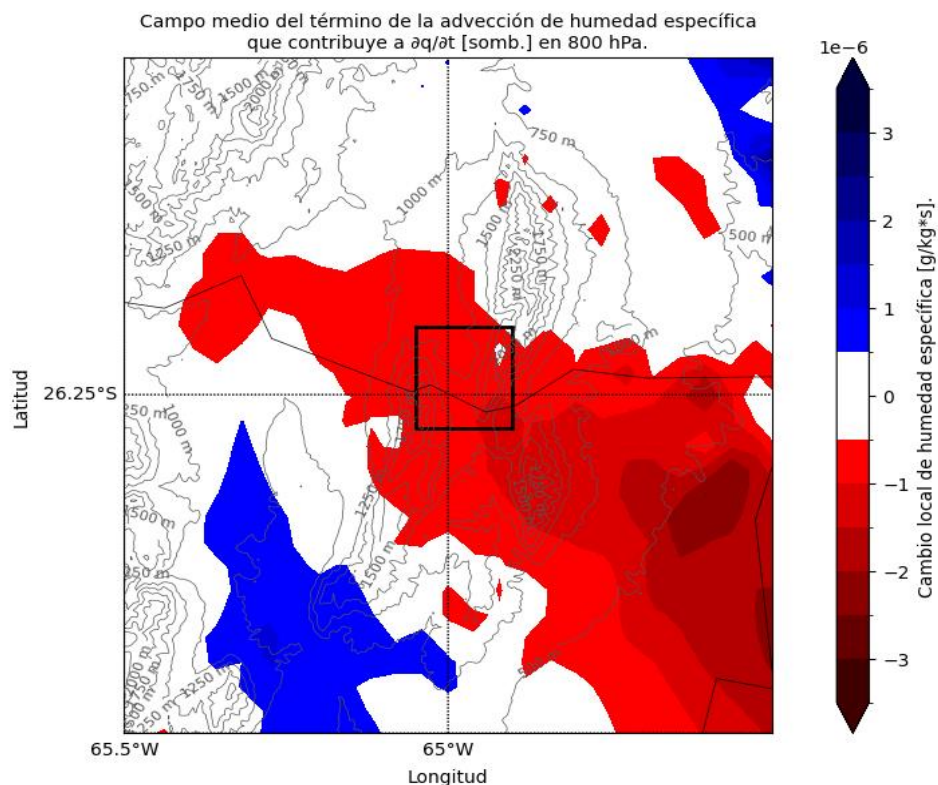
Fig. 16. Campo medio de variación local de humedad específica debido a advección de humedad en 800 hPa en días en que verifica el criterio propuesto de tormenta en el valle. Rectángulo negro: valle de interés.
