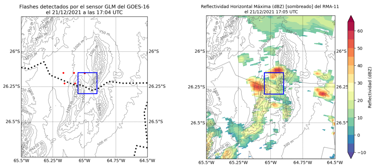
Fig. 4: Izq.: Mapeo de flashes (puntos rojos) del sensor GLM del GOES-16 sobre el valle de interés (rectángulo azul) para el día 21 de diciembre de 2021 a las 17:04 UTC. Der.: Imagen de reflectividad horizontal máxima del RMA-11 del 21 de diciembre de 2021 a las 17:05 UTC.
