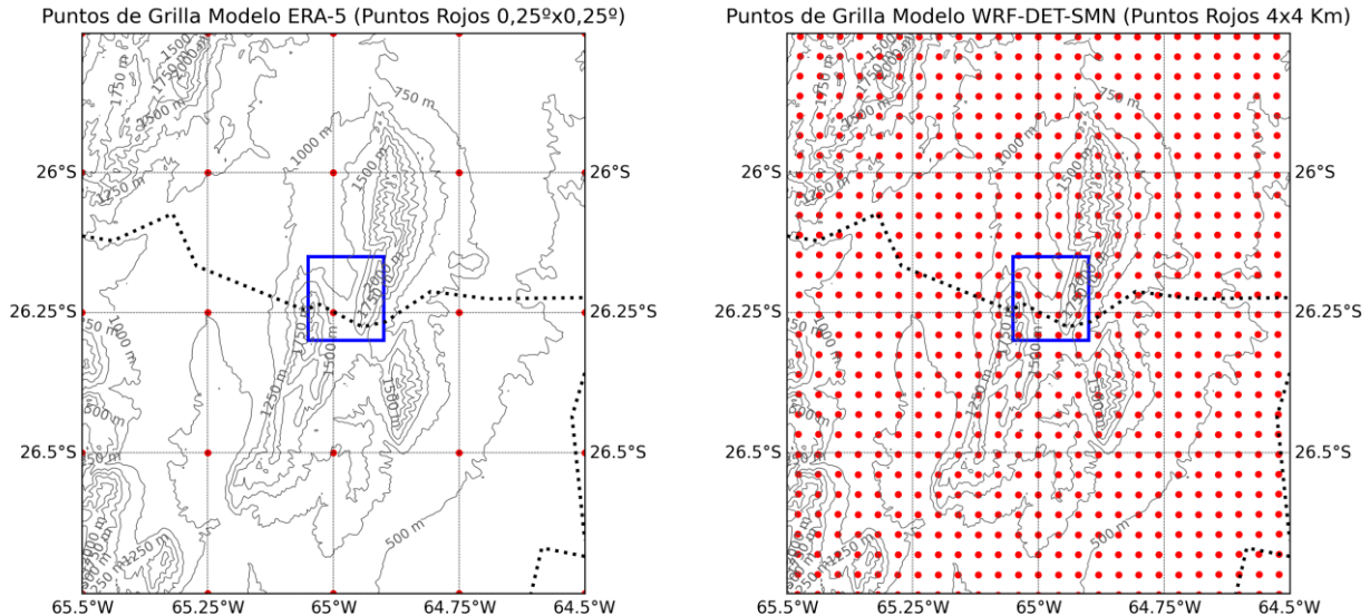
Fig. 7: Puntos de grilla para: a) modelo ERA-5 del centro Europeo. b) modelo WRF-SMN. El rectángulo azul identifica los bordes del valle de interés.
