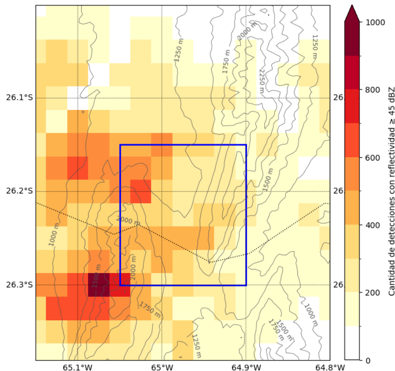
Fig. 10: Distribución espacial de volúmenes de muestreo con reflectividad \geq 45 dBZ identificados por el RMA-11, en casos que cumplen con el criterio de detección propuesto en el valle. Los colores representan la cantidad de detecciones en cada cuadrante, con una mayor concentración de eventos en las zonas en tonalidades más oscuras. El recuadro azul indica la región de interés analizada en el estudio.
