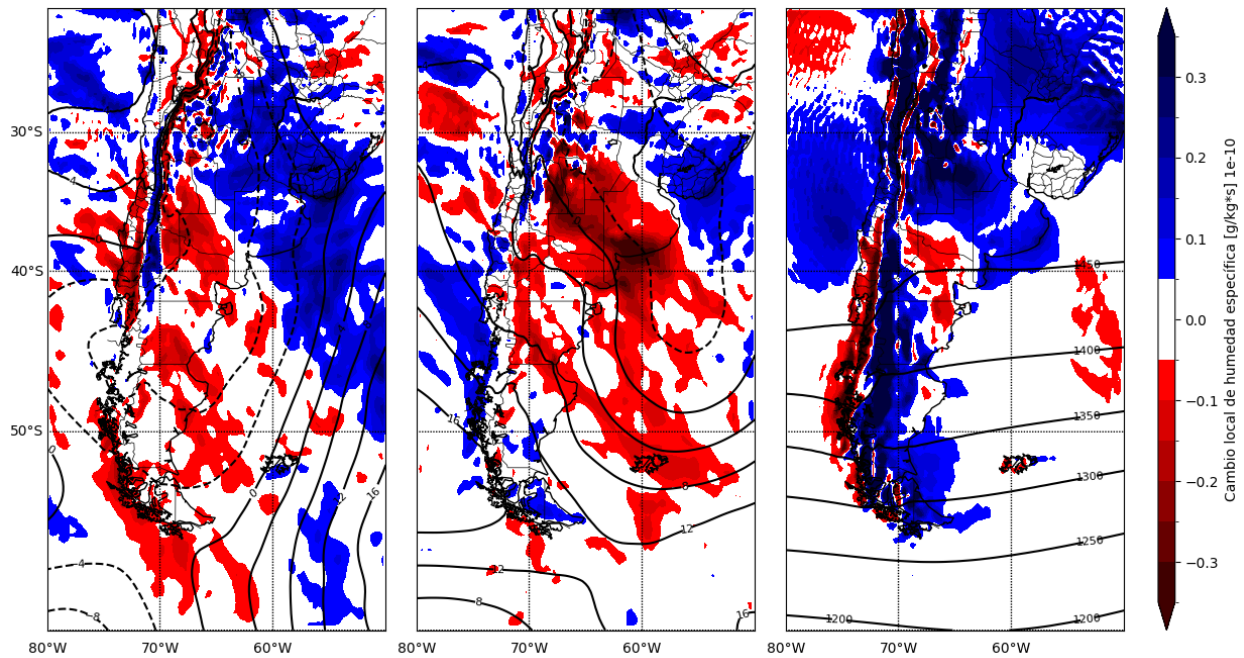
Fig. 13: Anomalías de tasa local de humedad específica por advección y de altura geopotencial en 850 hPa. Izq.: considerando el valor medio diario en el día previo en los que se identificó tormenta eléctrica según criterio propuesto; Centro: considerando el valor medio diario en el día en los que se identificó tormenta eléctrica según criterio, Der.: Tasa local de humedad específica por advección y altura geopotencial en 850 hPa climatológico.
