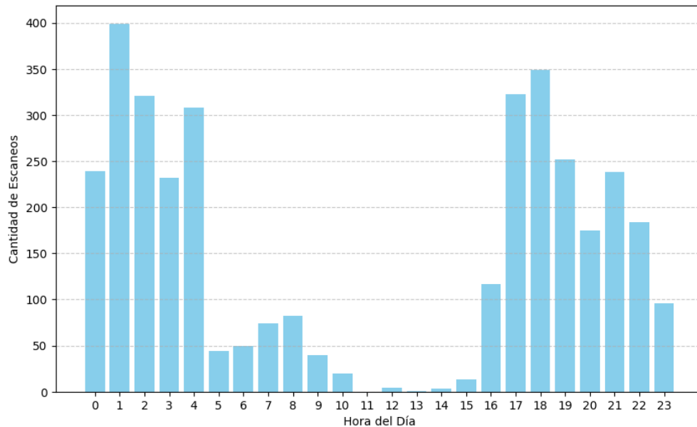
Fig. 8: Distribución horaria de los mapeos con detección en el valle consistidos con Z \geq 45 dBZ.
