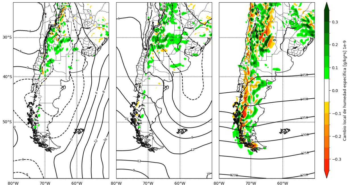
Fig. 14: Anomalías de tasa local de humedad específica por convergencia y de altura geopotencial en 850 hPa. Izquierda: considerando el valor medio diario en el día previo en los que se identificó tormenta eléctrica según criterio propuesto; Centro: considerando el valor medio diario en el día en los que se identificó tormenta eléctrica según criterio, Derecha: Tasa local de humedad específica por convergencia y altura geopotencial en 850 hPa climatológico.
