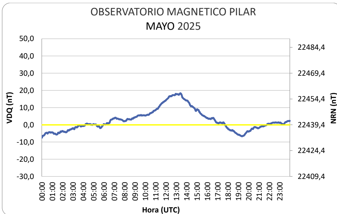
Figura 8: Variación Diaria Calma del mes de mayo
