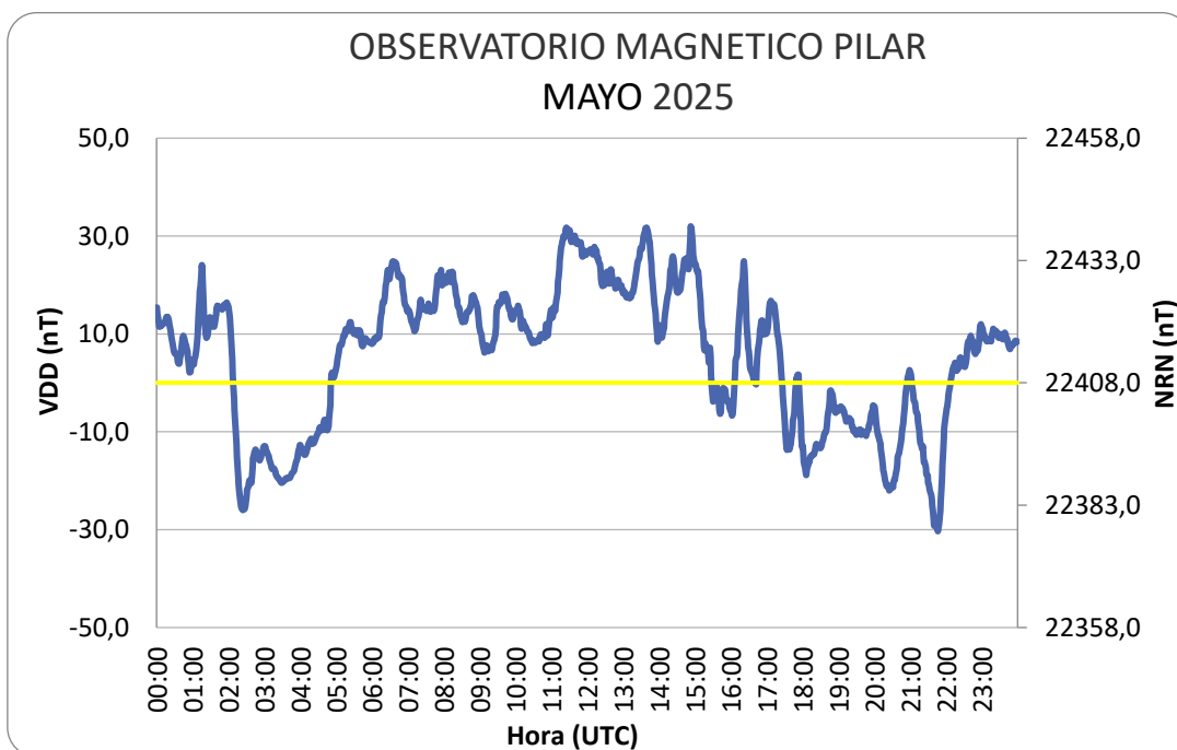
Figura 9: Variación Diaria Perturbada del mes de mayo
