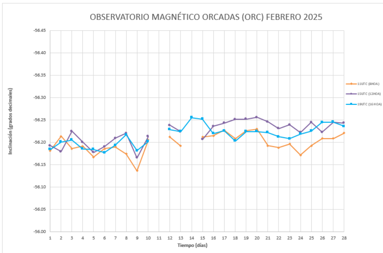
Figura 6: Inclinación magnética en función del tiempo
