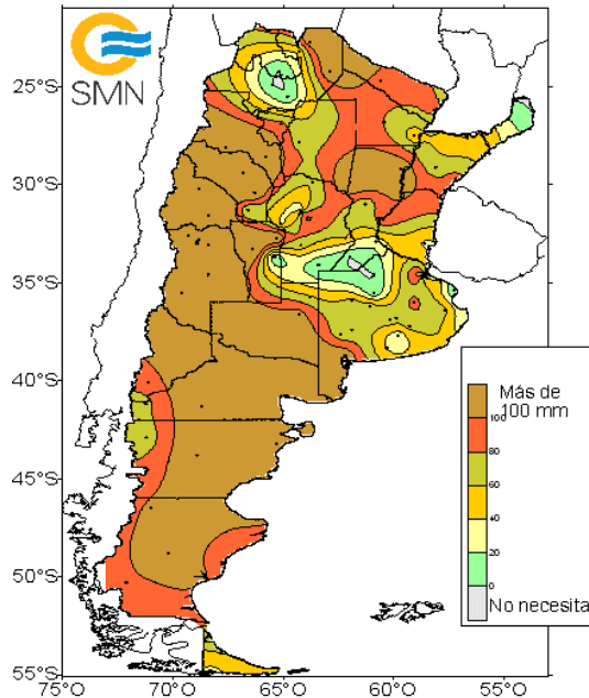
Agua necesaria para no estar en Sequía en los próximos 10 días a partir del 10 de febrero de 2025
