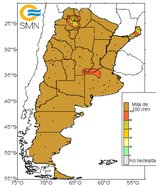
Agua necesaria para comenzar a tener Excesos en los próximos 10 días a partir del 10 de febrero de 2025
