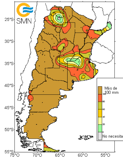
Agua necesaria para no estar en Comienzo de Sequía en los próximos 10 días a partir del 10 de febrero de 2025
