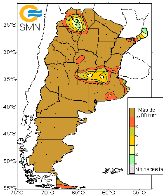
Agua necesaria para tener Buenas Condiciones en los próximos 10 días a partir del 10 de febrero de 2025
