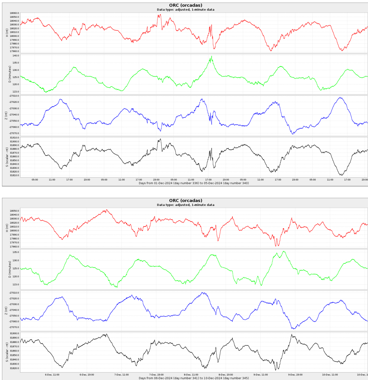
Figura 4a: Componentes del campo magnético del 1 al 10 de diciembre. En rojo se ve la componente horizontal (H) y en azul la vertical (Z), ambas en nT. En verde se presenta la declinación del campo magnético (D) en minutos y en negro la intensidad del campo magnético en nT
