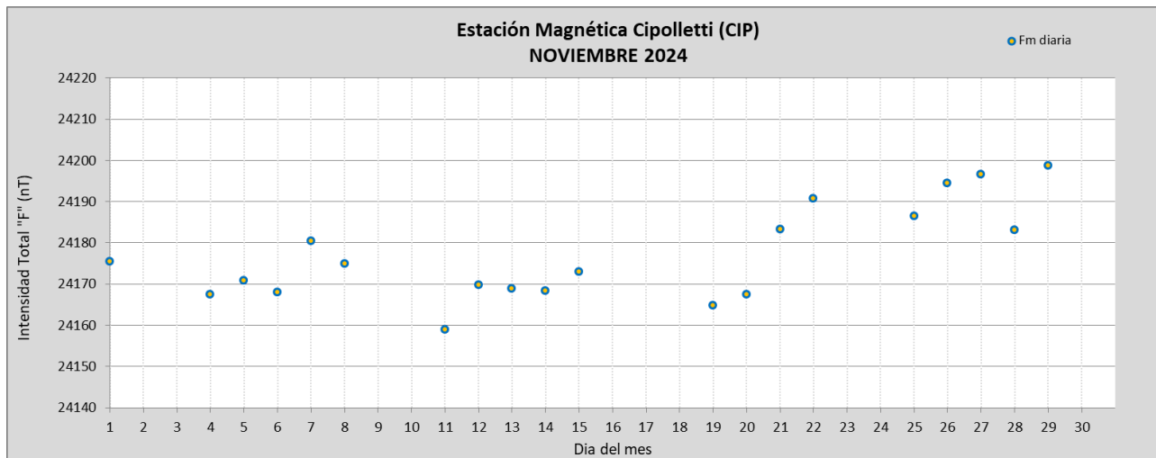
Figuras 5: Intensidad total del campo magnético en función del tiempo
