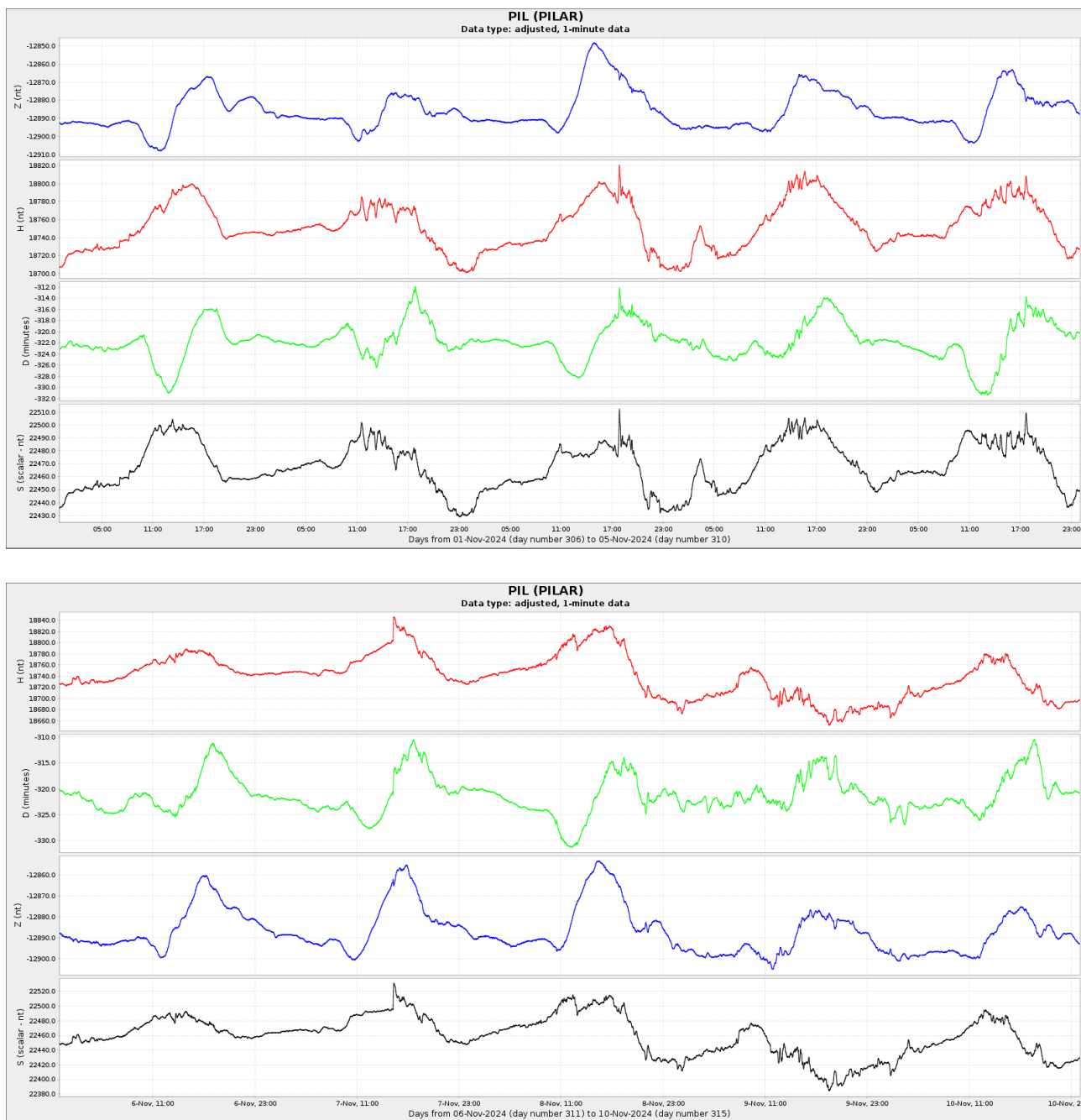
Figura 4a: Componentes del campo magnético del día 1 al 10 de noviembre. En rojo se ve la componente horizontal ( H ) y en azul la vertical ( Z ), ambas en nT. En verde se presenta la declinación del campo magnético ( D ) en minutos y en negro la intensidad del campo magnético en nT.
