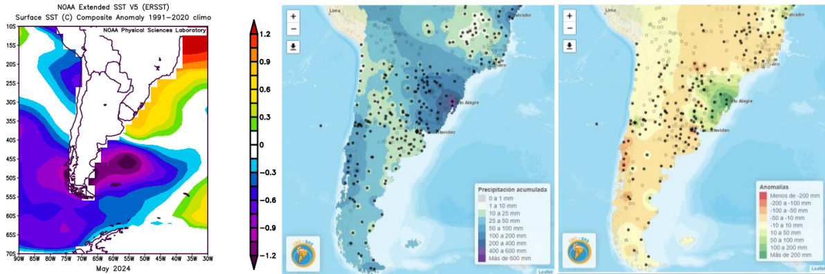
FIG. 8 –Anomalías de la temperatura superficial del mar de mayo de 2024. Período de referencia 1991-2020. Fuente: NOAA. Precipitación acumulada (centro) y anomalía (derecha) (mm) – mayo de 2024– Fuente: CRC-SAS
