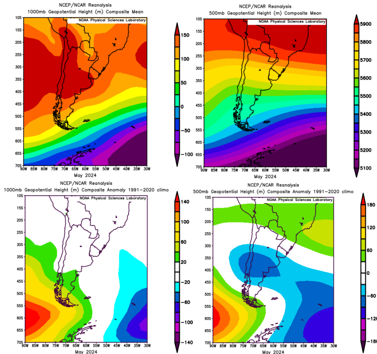
FIG.7- Campo medio de altura geopotencial de la superficie isobárica de 1000 y 500 hPa (arriba) (m) y anomalía (abajo) mayo de 2024
