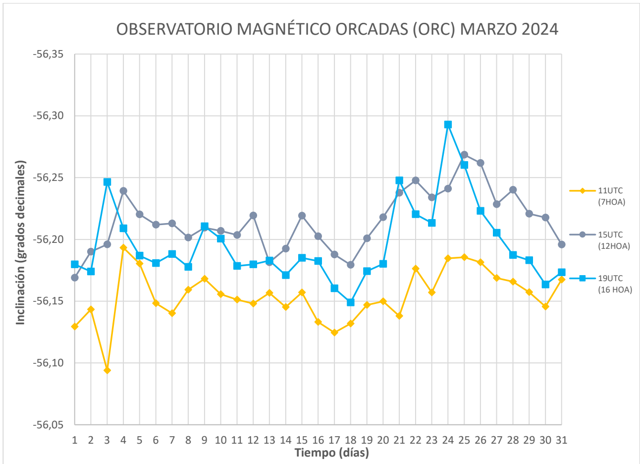
Figura 6: Inclinación magnética en función del tiempo
