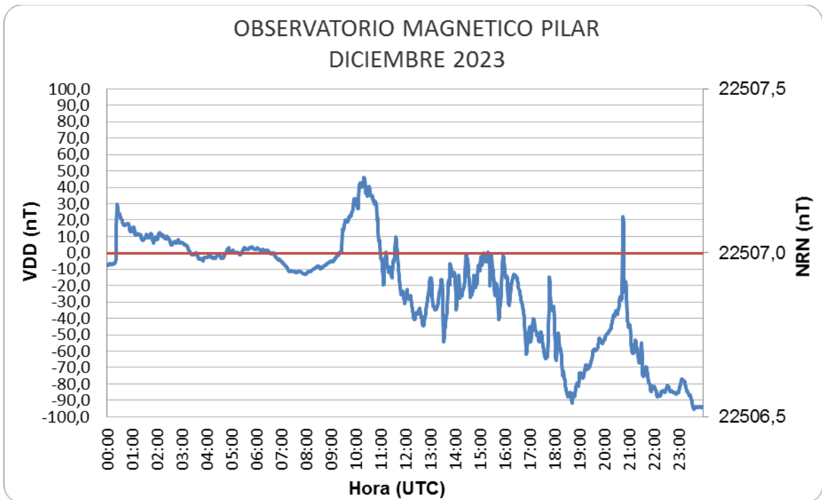
Figura 9: Variación Diaria Perturbada del mes de Diciembre
