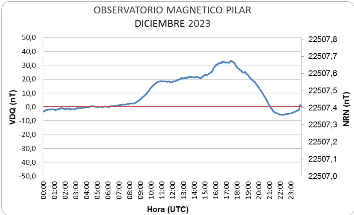
Figura 8: Variación Diaria Calma del mes de Diciembre
