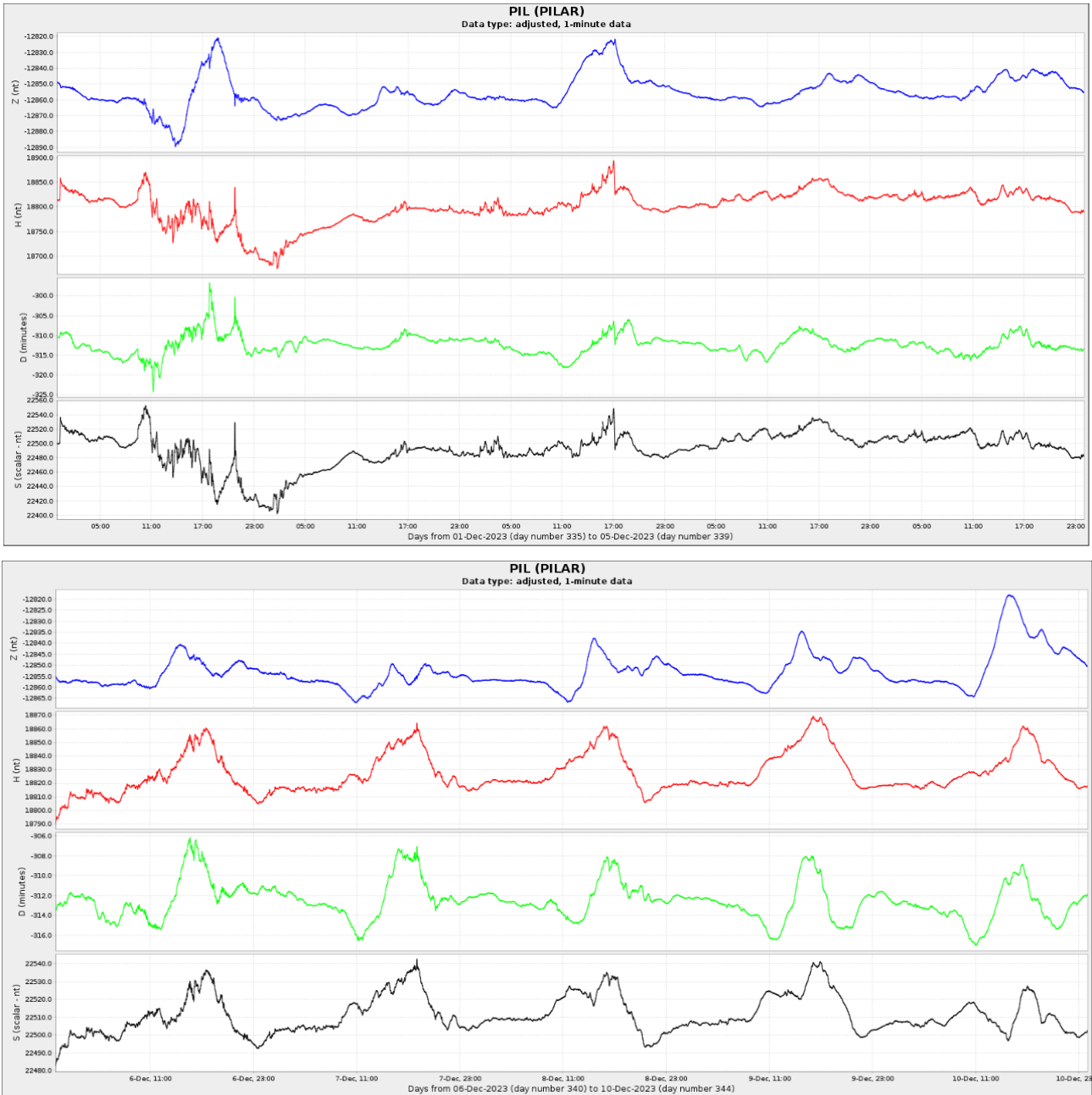
Figura 4a: Componentes del campo magnético del día 1 al 10 de diciembre. En rojo se ve la componente horizontal (H) y en azul la vertical (Z), ambas en nT. En verde se presenta la declinación del campo magnético (D) en minutos y en negro la intensidad del campo magnético en nT.
