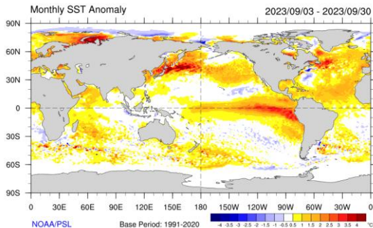
Figura 1 - Anomalías de la temperatura superficial del mar de septiembre de 2023. Período de referencia 1991-2020. Fuente: NOAA-CIRES/CDC
