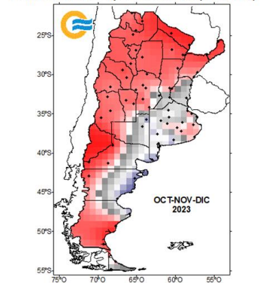
Pronóstico de Temperatura Media (Modelo 1)
