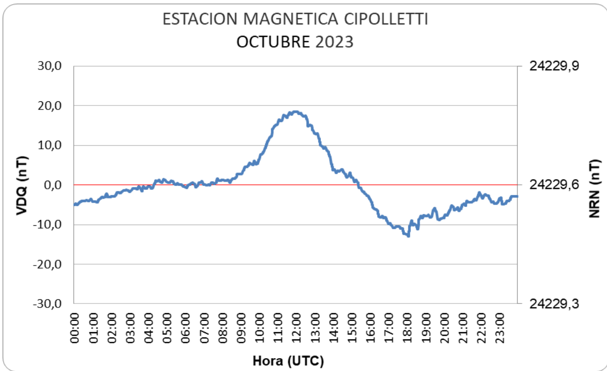
Figura 7: Variación Diaria Calma del mes de octubre
