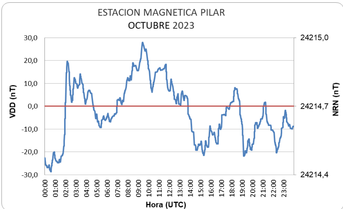
Figura 8: Variación Diaria Perturbada del mes de octubre
