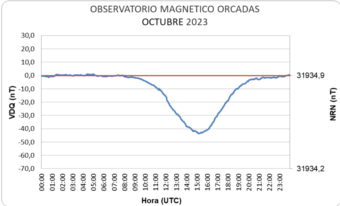
Figura 8: Variación Diaria Calma del mes de octubre
