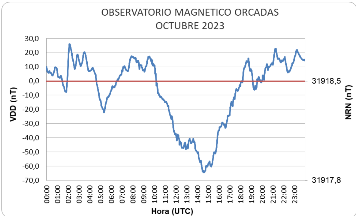
Figura 9: Variación Diaria Perturbada del mes de octubre
