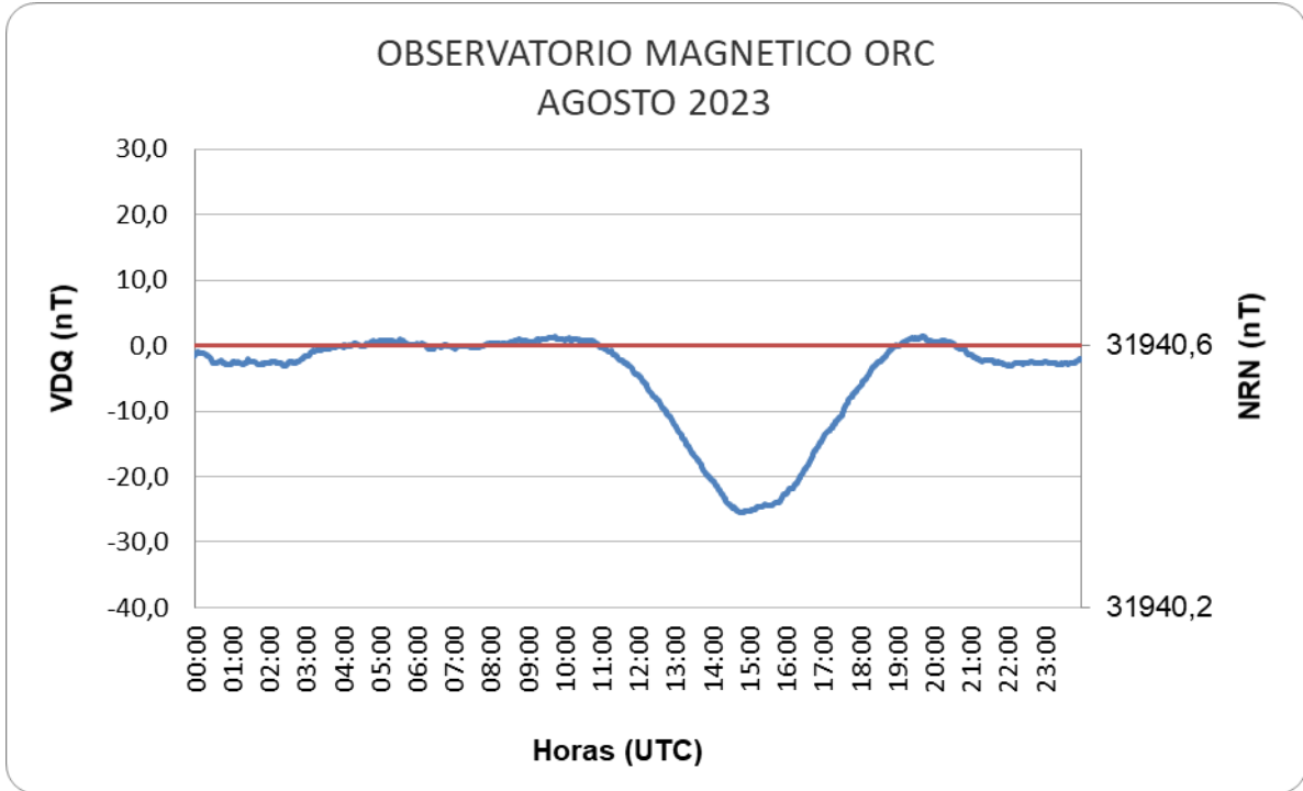
Figura 8: Variación Diaria Calma del mes de agosto
