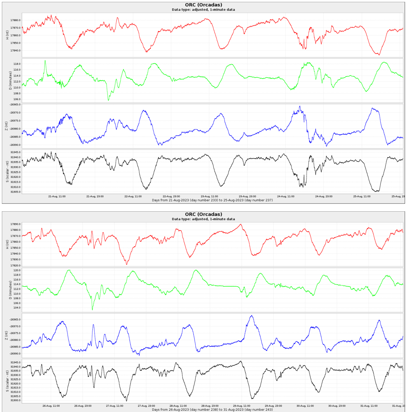
Figura 4c: Componentes del campo magnético del 21 al 31 de agosto. En rojo se ve la componente horizontal (H) y en azul la vertical (Z), ambas en nT. En verde se presenta la declinación del campo magnético (D) en minutos y en negro la intensidad del campo magnético en nT.
