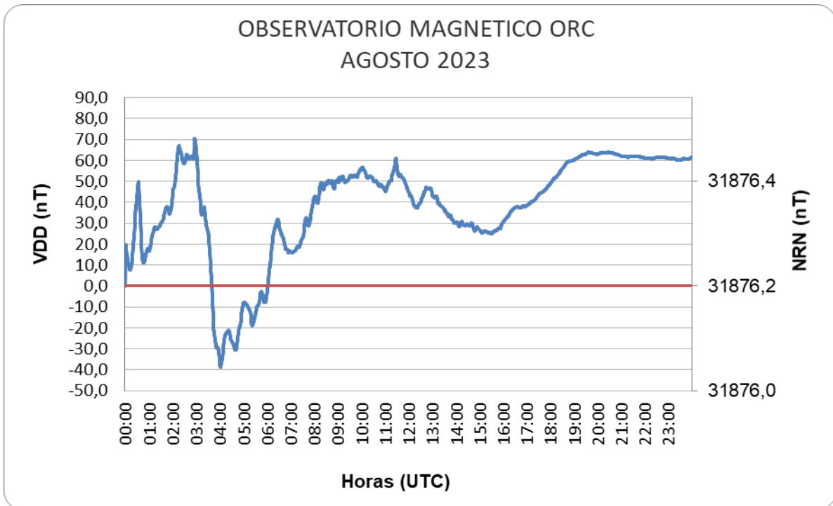
Figura 9: Variación Diaria Perturbada del mes de agosto
