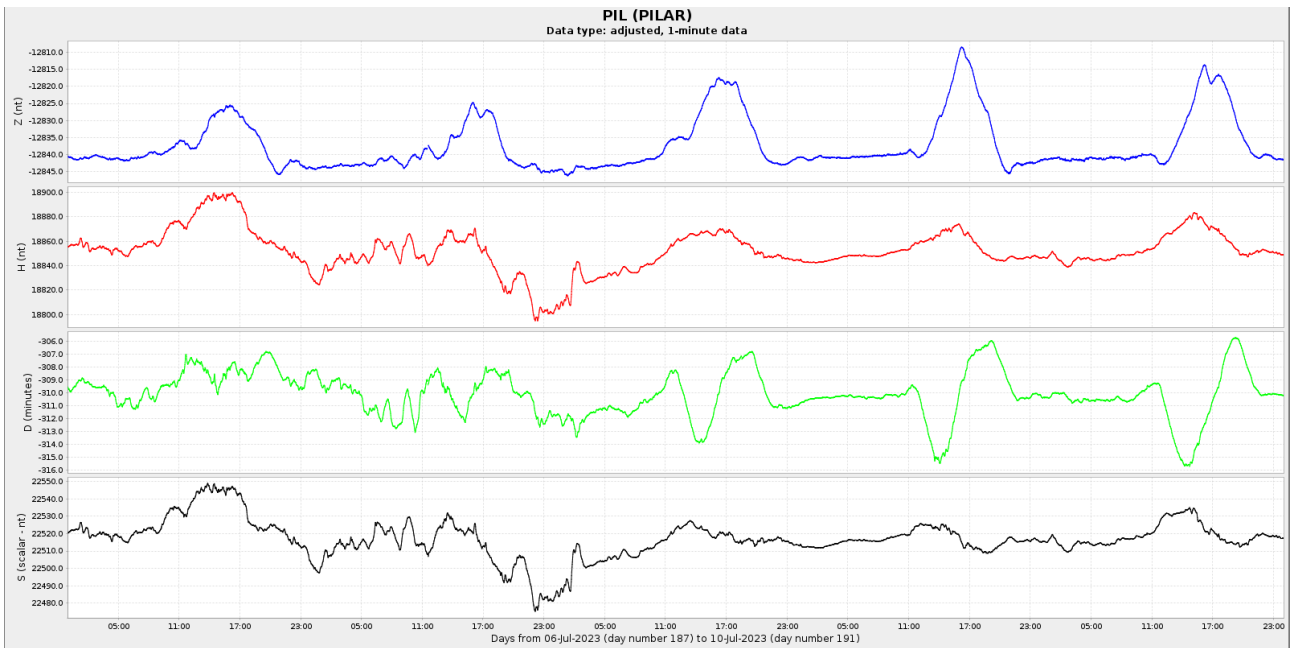
Figura 4a: Componentes del campo magnético del día 1 al 10 de julio. En rojo se ve la componente horizontal (H) y en azul la vertical (Z), ambas en nT. En verde se presenta la declinación del campo magnético (D) en minutos y en negro la intensidad del campo magnético en nT.
