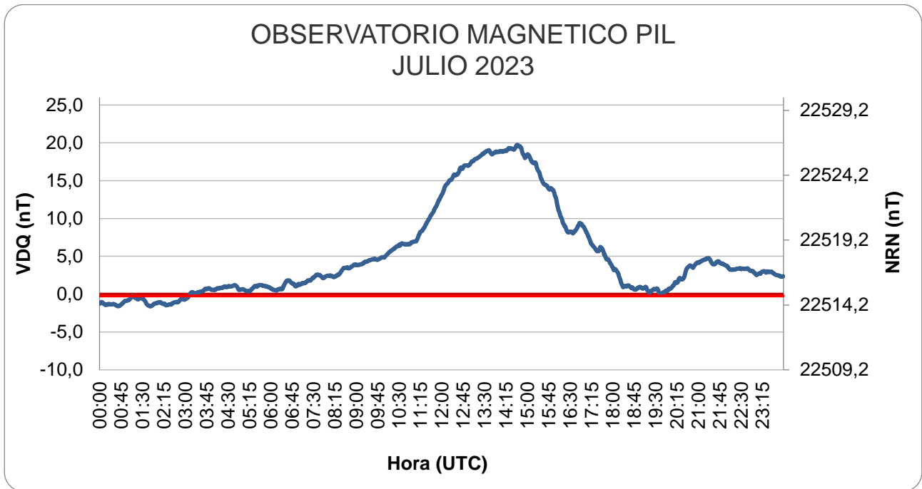
Figura 8: Variación Diaria Calma del mes de julio
