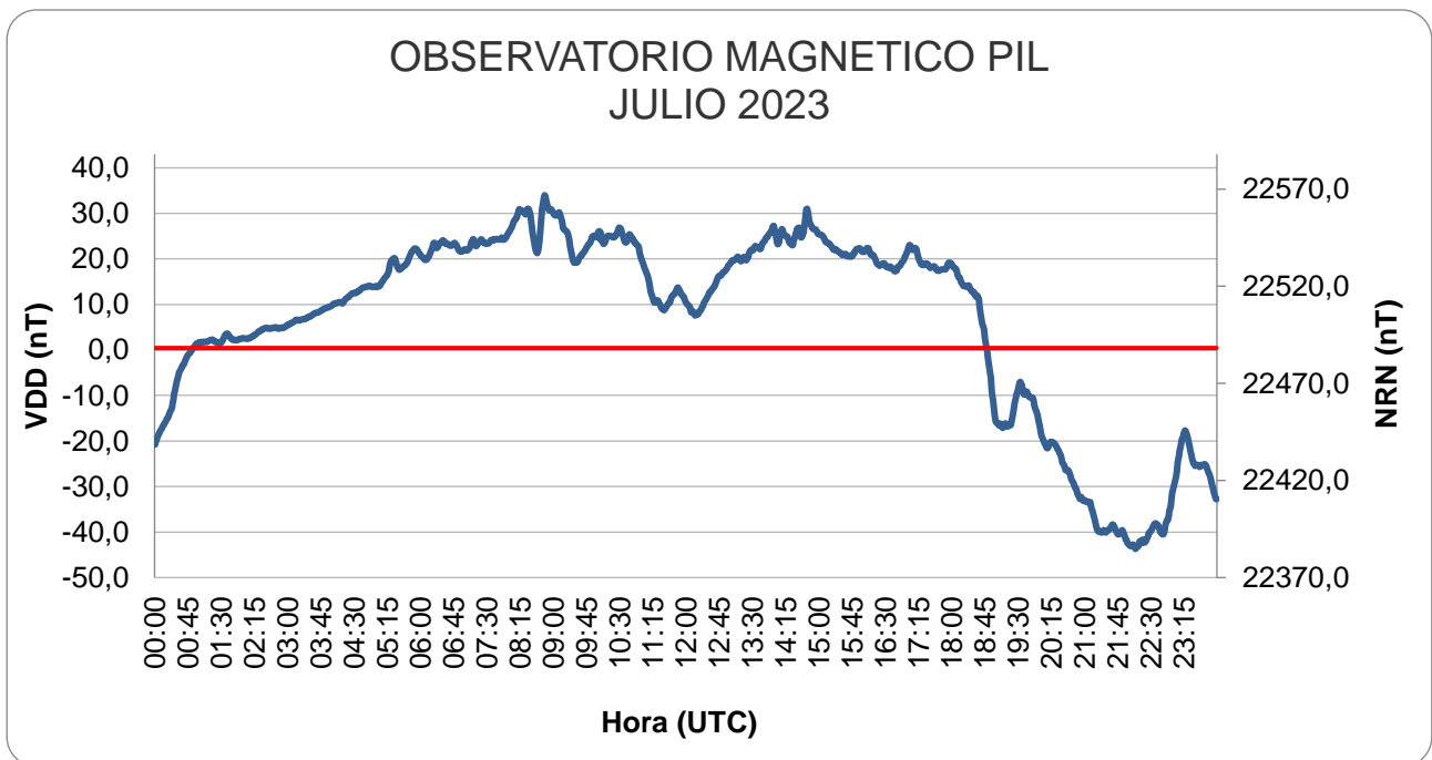
Figura 9: Variación Diaria Perturbada del mes de julio
