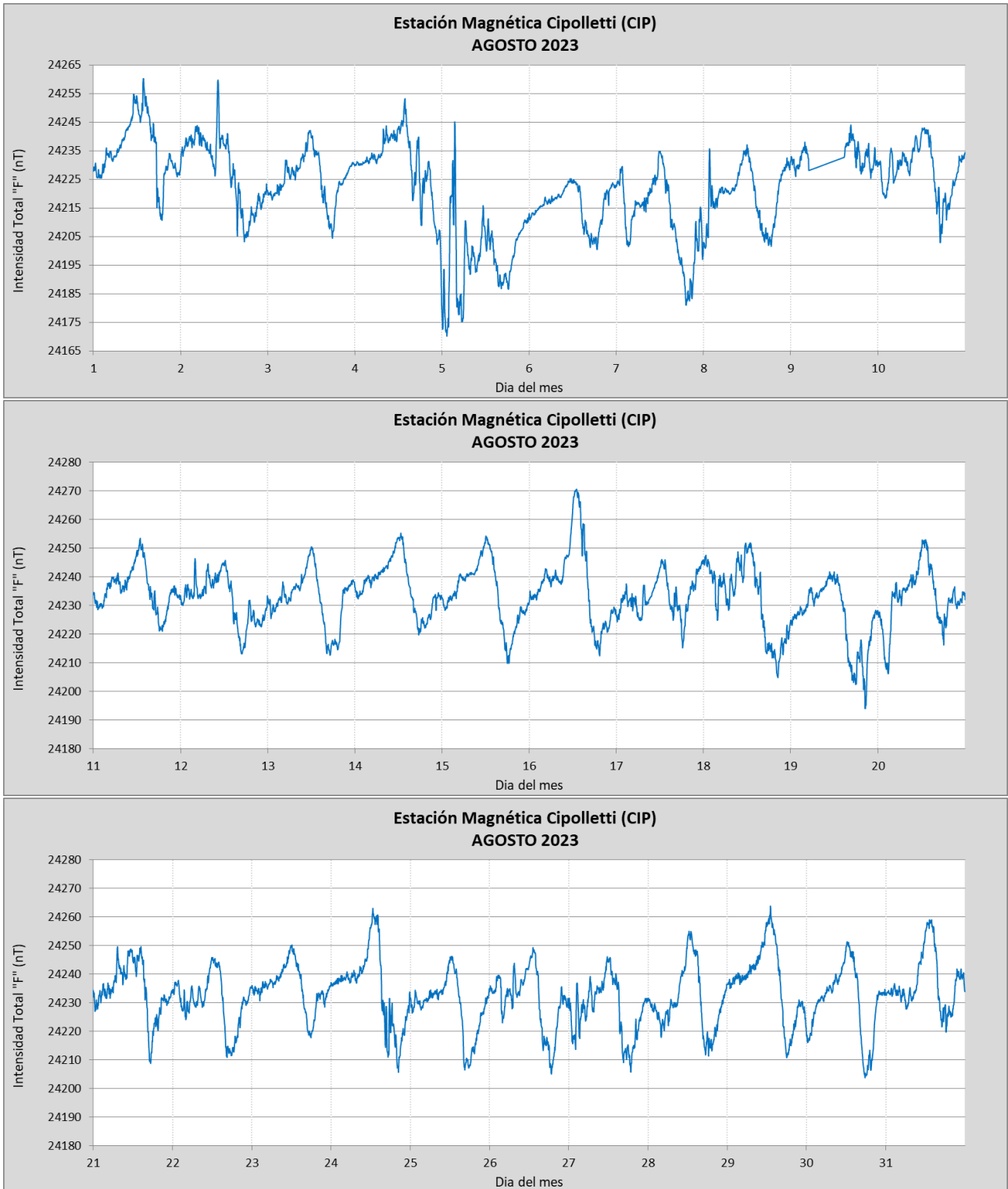
Figuras 5 (a,b,c): Intensidad total del campo magnético en función del tiempo
