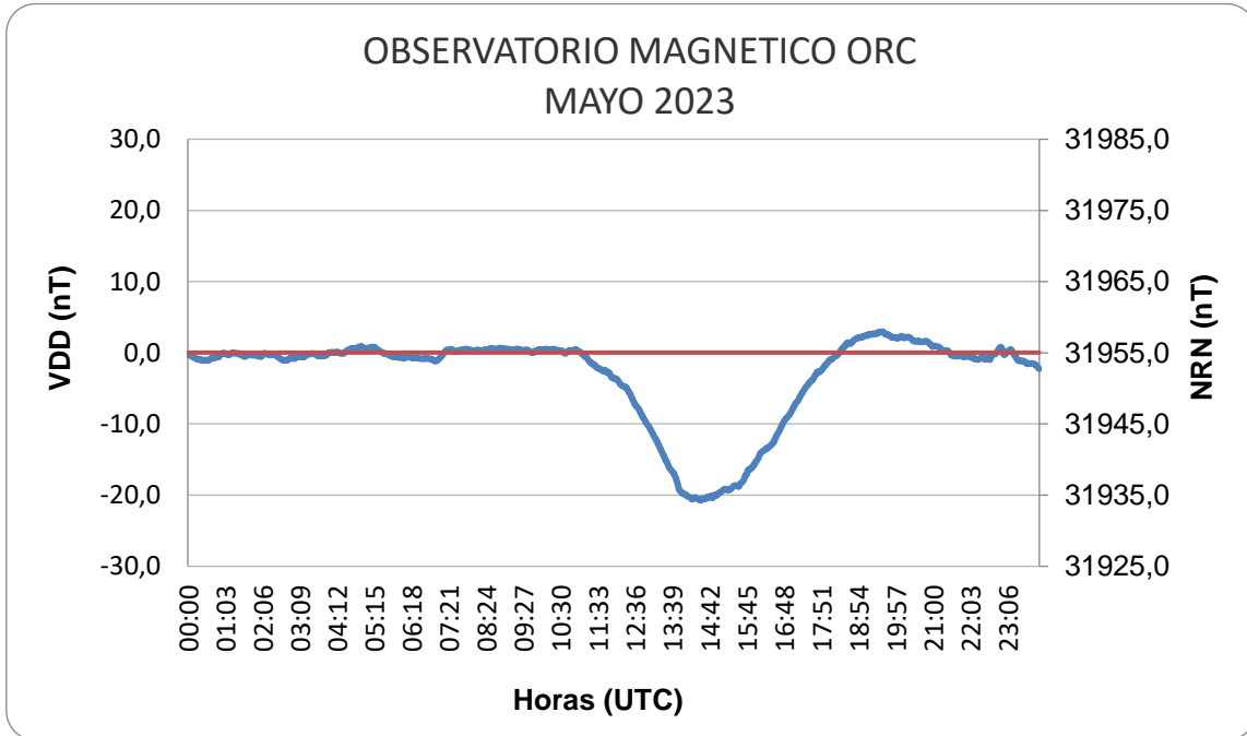
Figura 8: Variación Diaria Calma del mes de mayo
