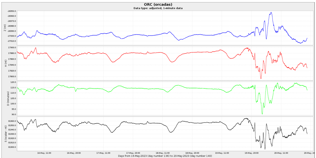
Figura 4b Componentes del campo magnético del 11 al 20 de mayo. En rojo se ve la componente horizontal (H) y en azul la vertical (Z), ambas en nT. En verde se presenta la declinación del campo magnético (D) en minutos y en negro la intensidad del campo magnético en nT.
