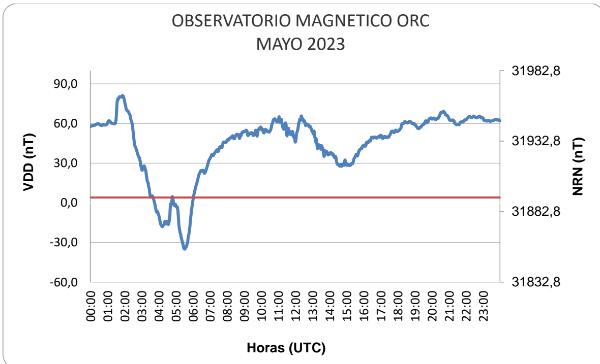
Figura 9: Variación Diaria Perturbada del mes de mayo
