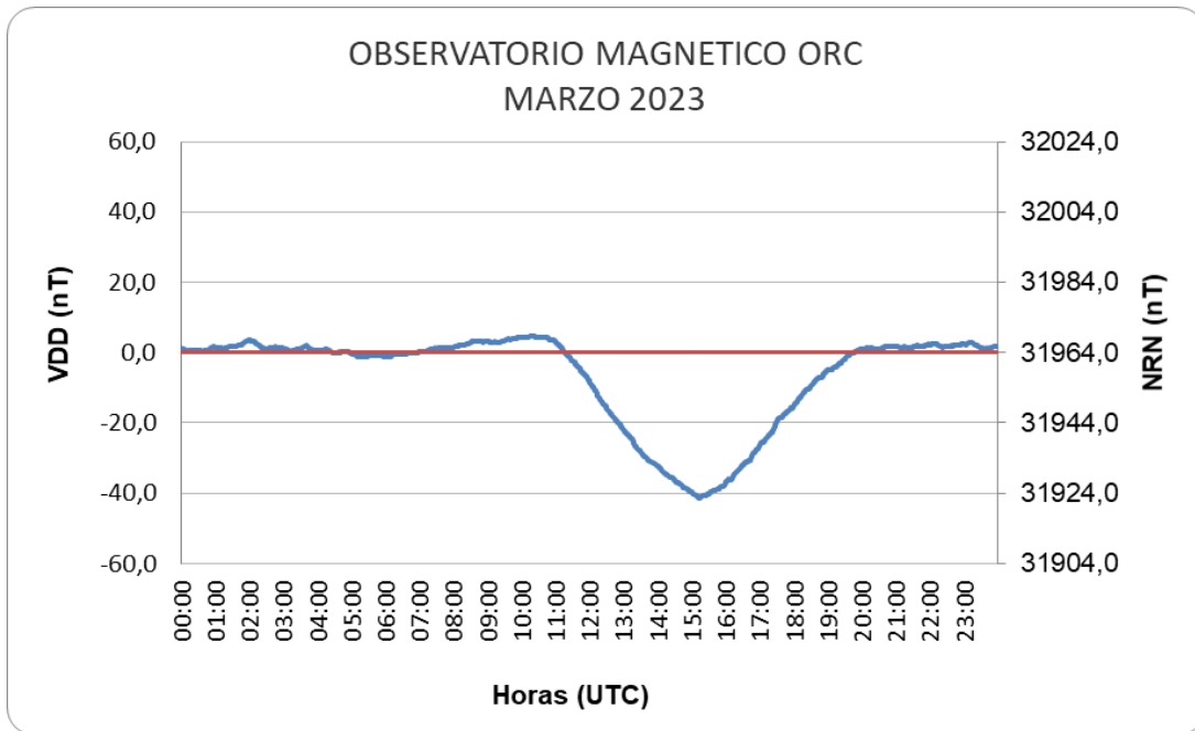
Figura 8: Variación Diaria Calma del mes de marzo
