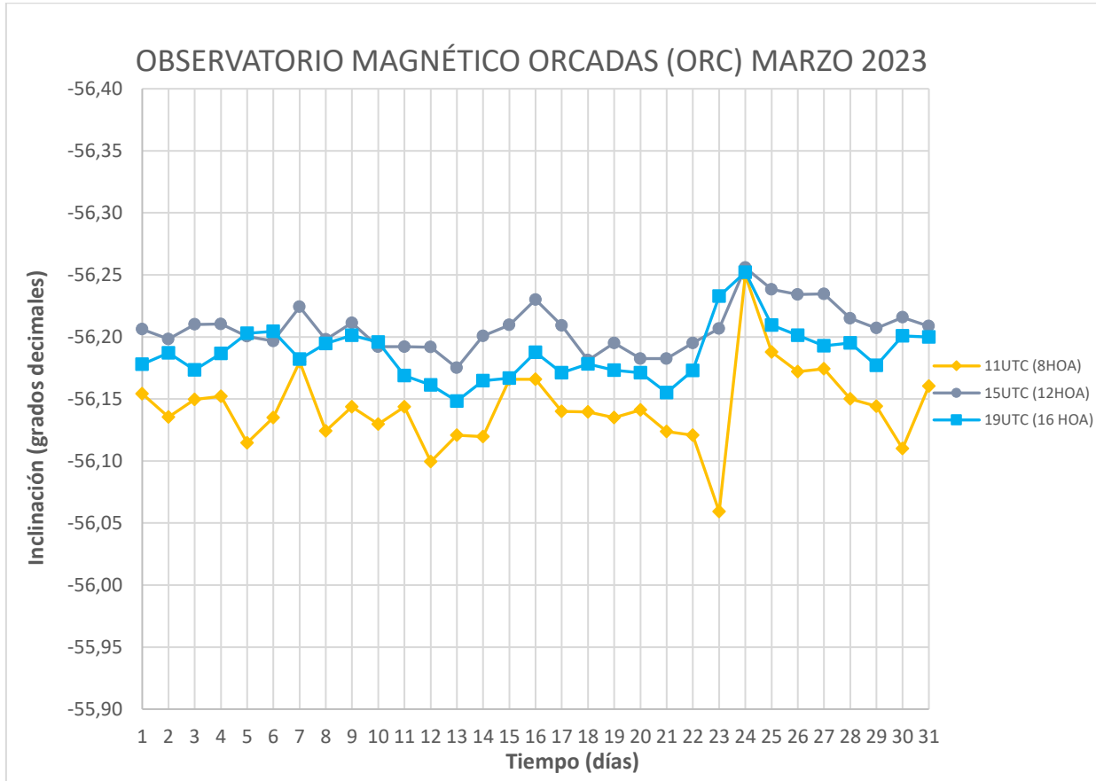
Figura 6: Inclínación magnética en función del tiempo
