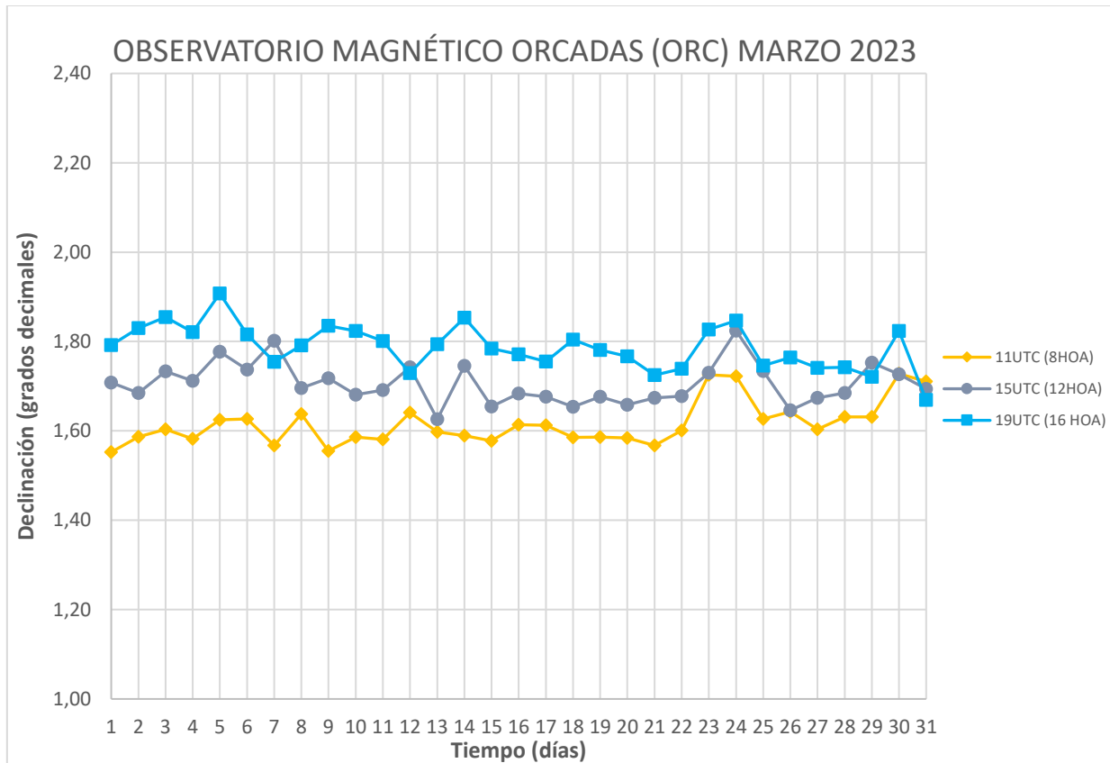
Figura 5: Declinación magnética en función del tiempo
